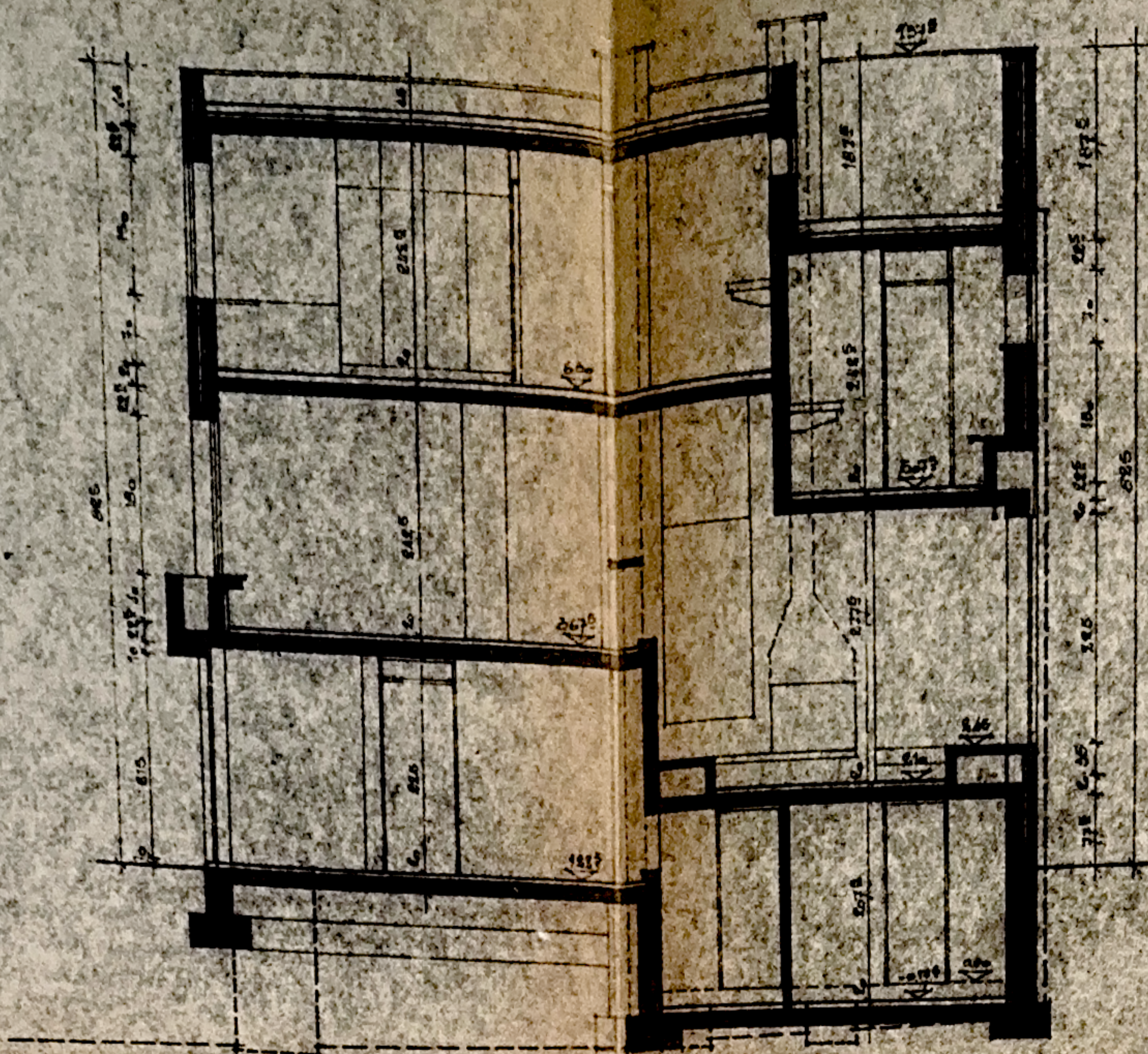
DOORSNEDE AA
