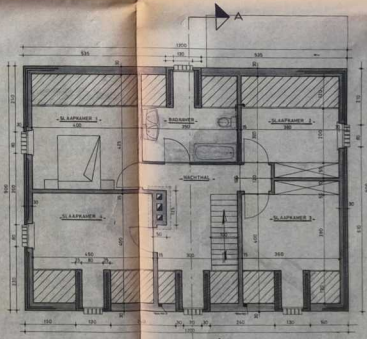
PLAN VERDIEP
