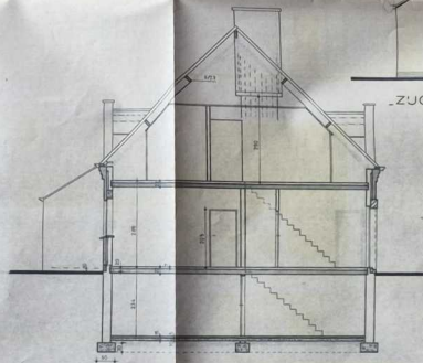
DOORSNEDE AA
