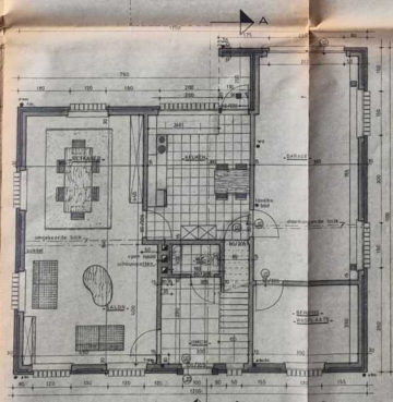
PLAN GELUKVLOERS
