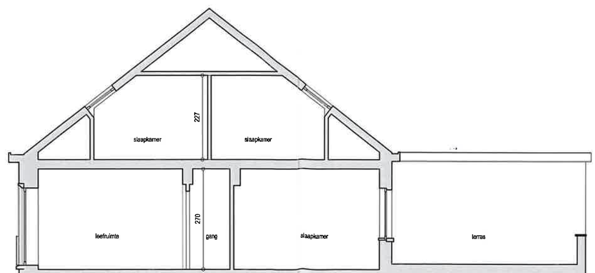
DOORSNEDE
