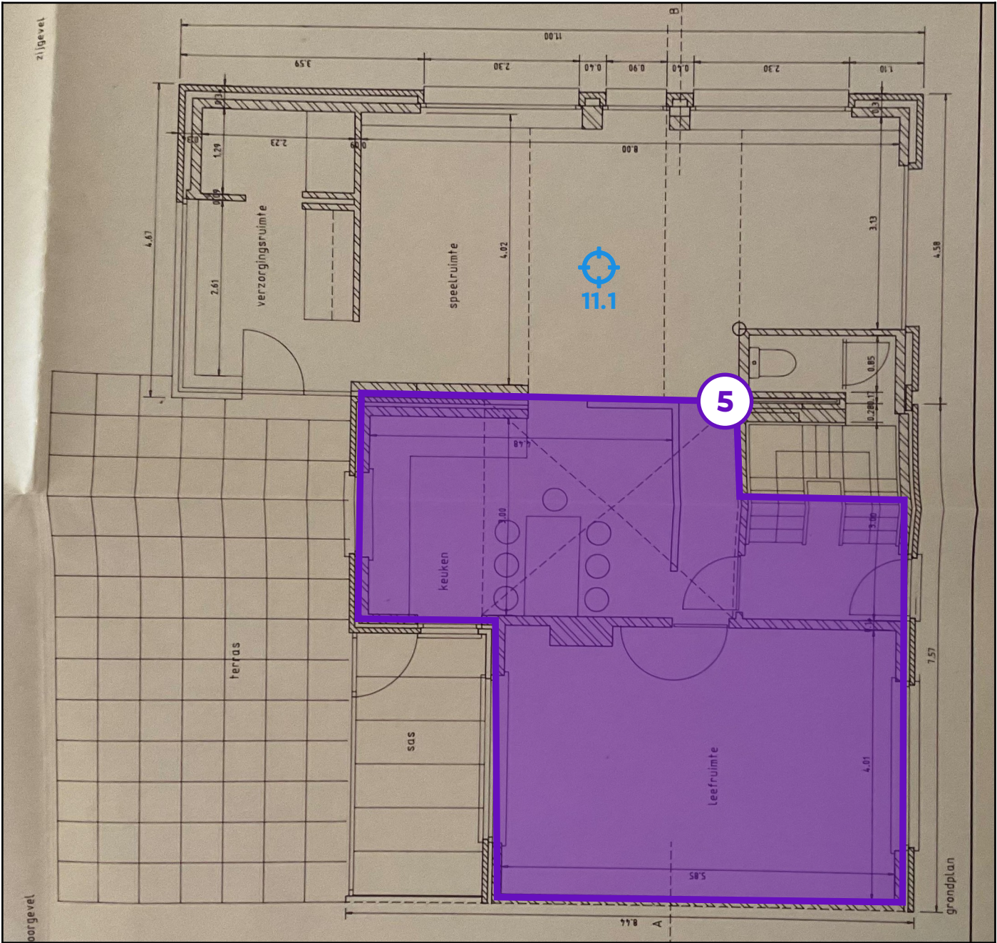
Legende van plan 1.6: Gelijkvloers (plafondpleister)
