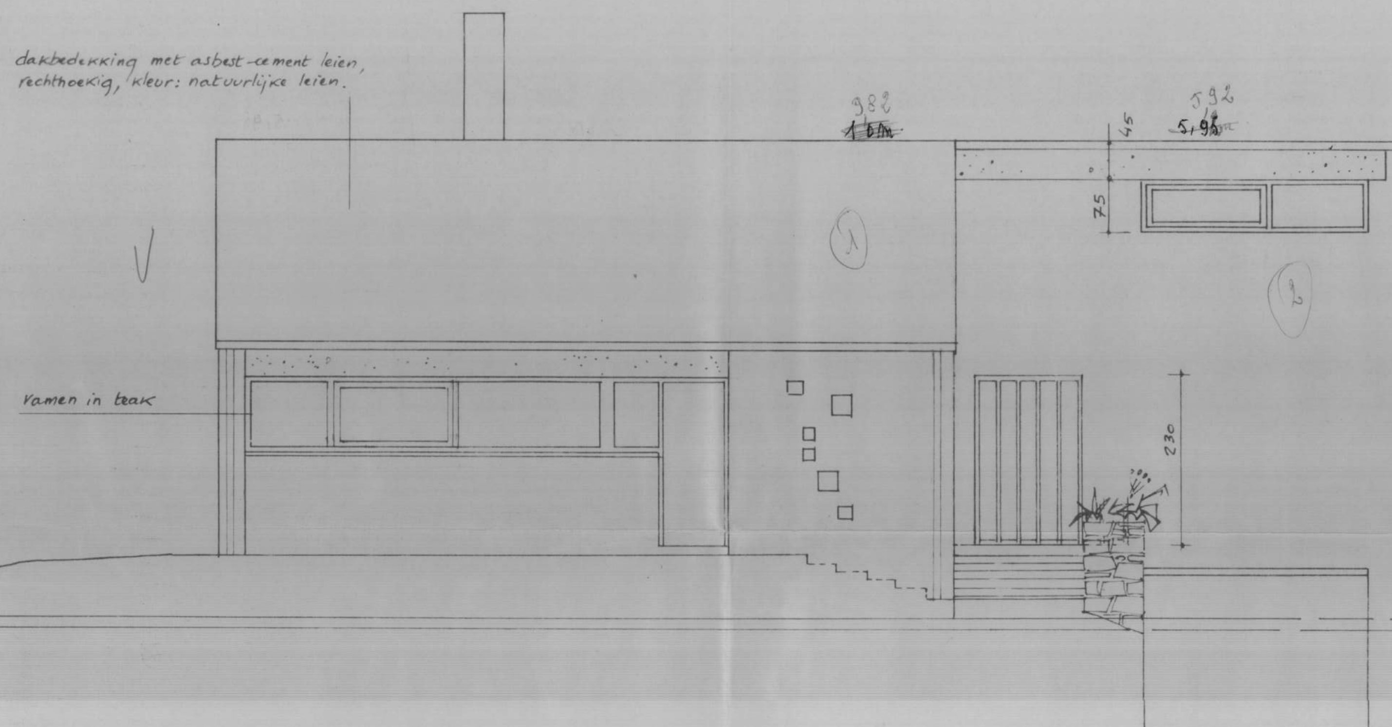
OOSTGEVEL
