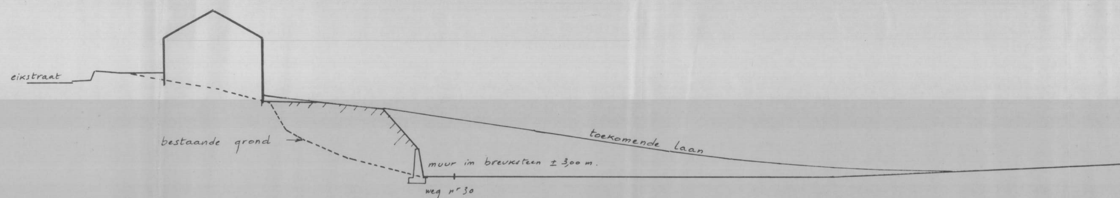
PROFIEL TERREIN EN TOEKOMENDE LAAN, SCHAAL 1/250
