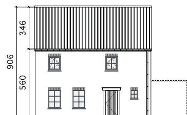
VOORGEVEL
