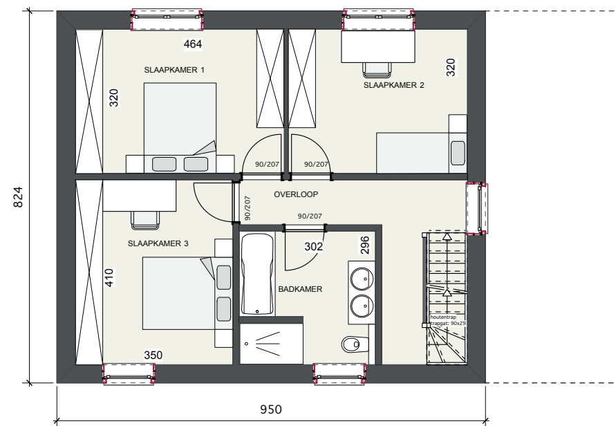
VERDIEPING
