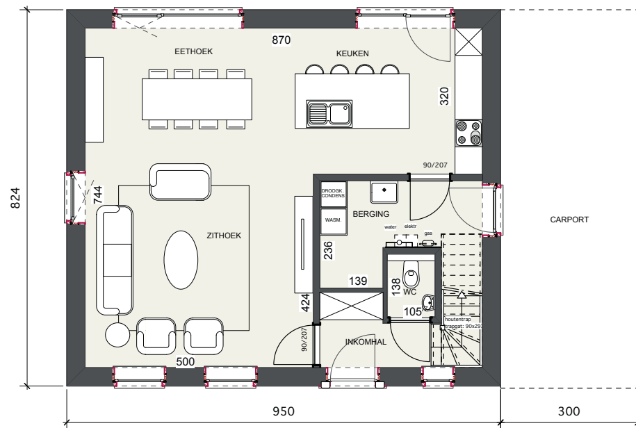
GELIJKVLOERS
