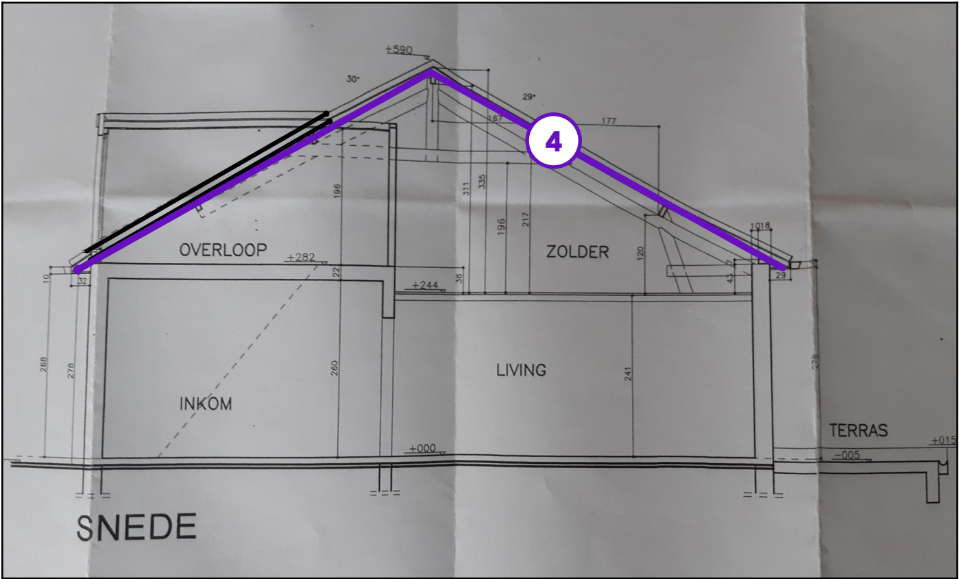
Legende van plan 1.5: Snede van het huis
