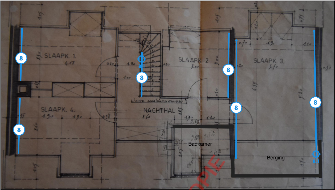
Legende van plan 1.4: Grondplan - 1ste verdieping
