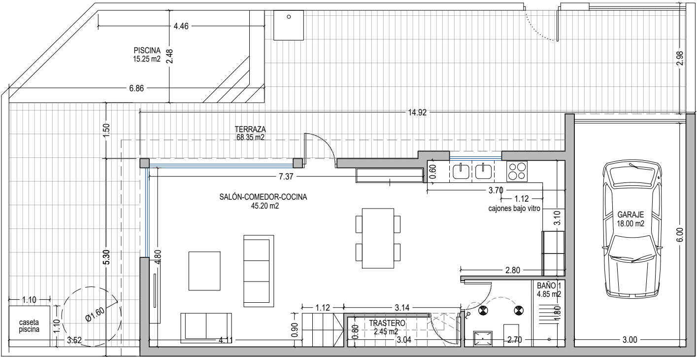
PLANTA BAJA
