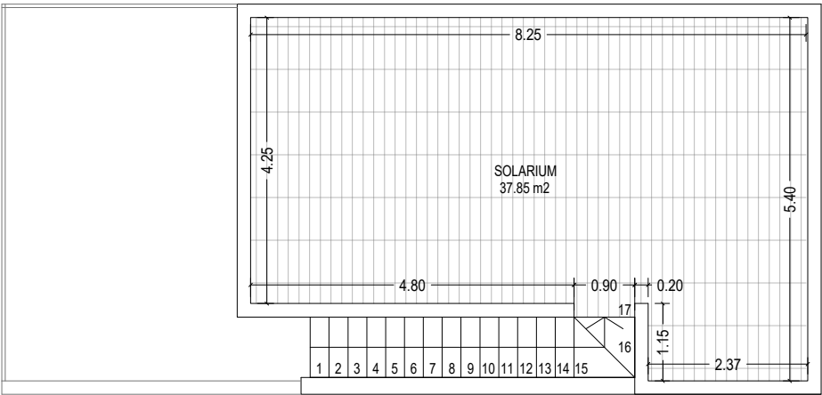
PLANTA CUBIERTA
