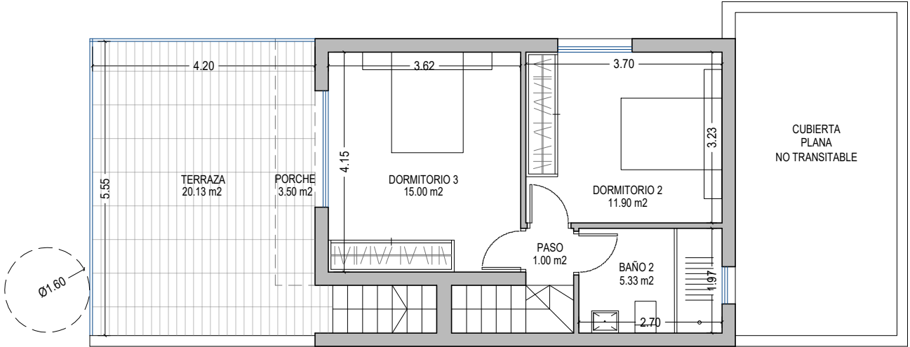
PLANTA PRIMERA
