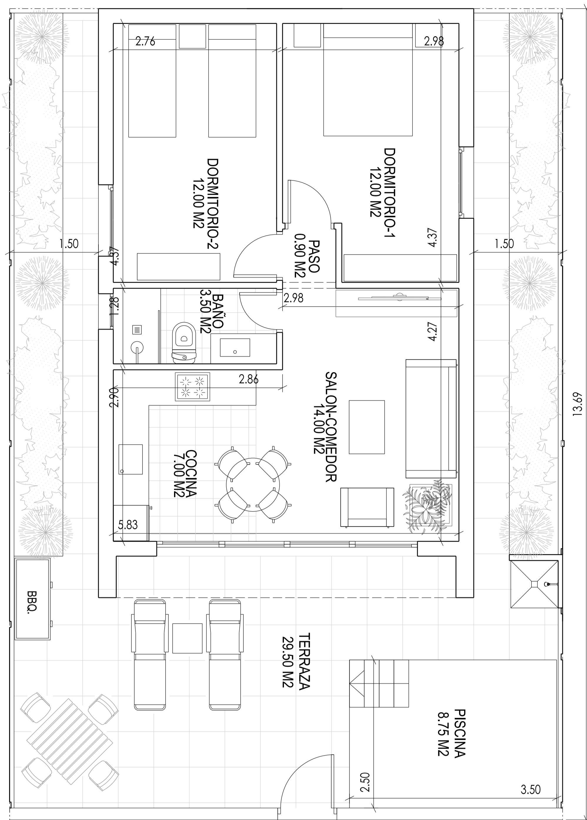
PLANTA BAJA
