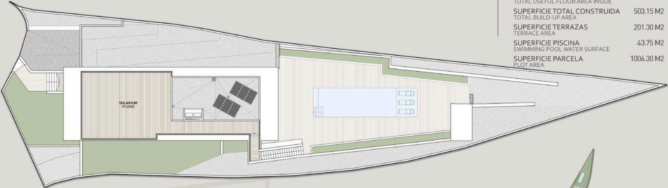
PLANTA SOLARIUM
