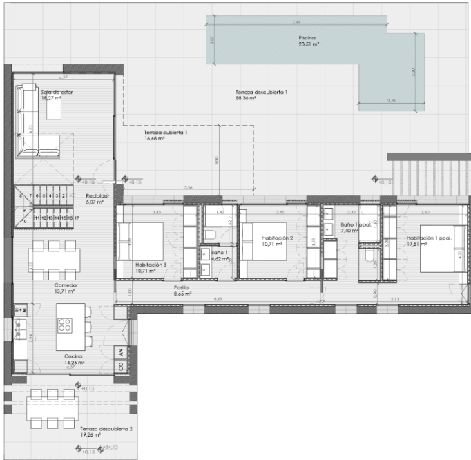
PLANTA BAJA 1:100
