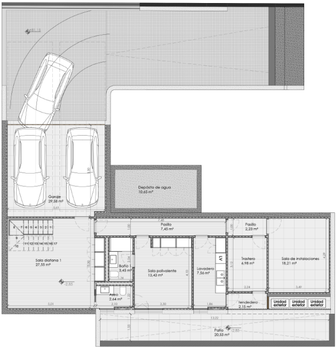
PLANTA SÓTANO 1:100
