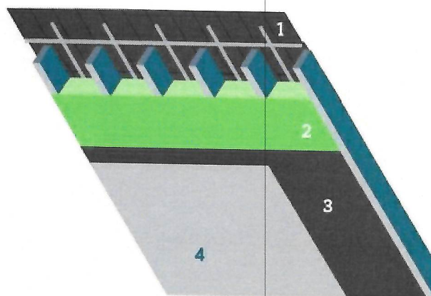
1. Onderdak | 2. Isolatatie | 3. Dampscherm | 4. binnenafwerking
