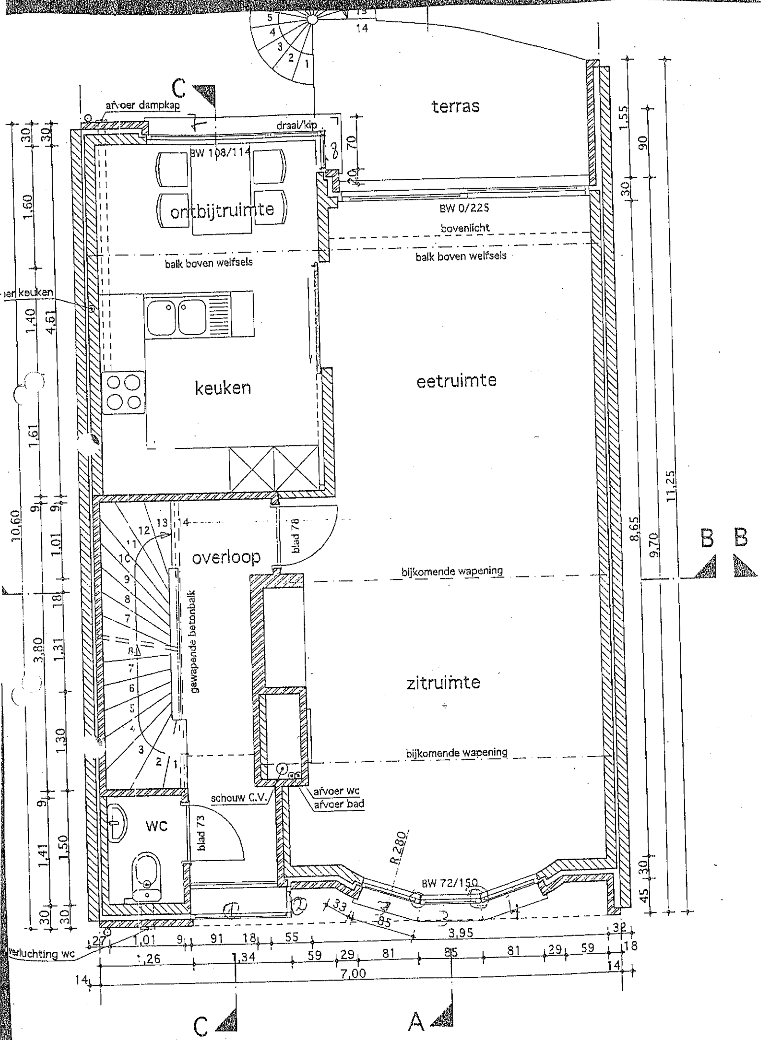
VERDIEPINGSPLAN - 1
