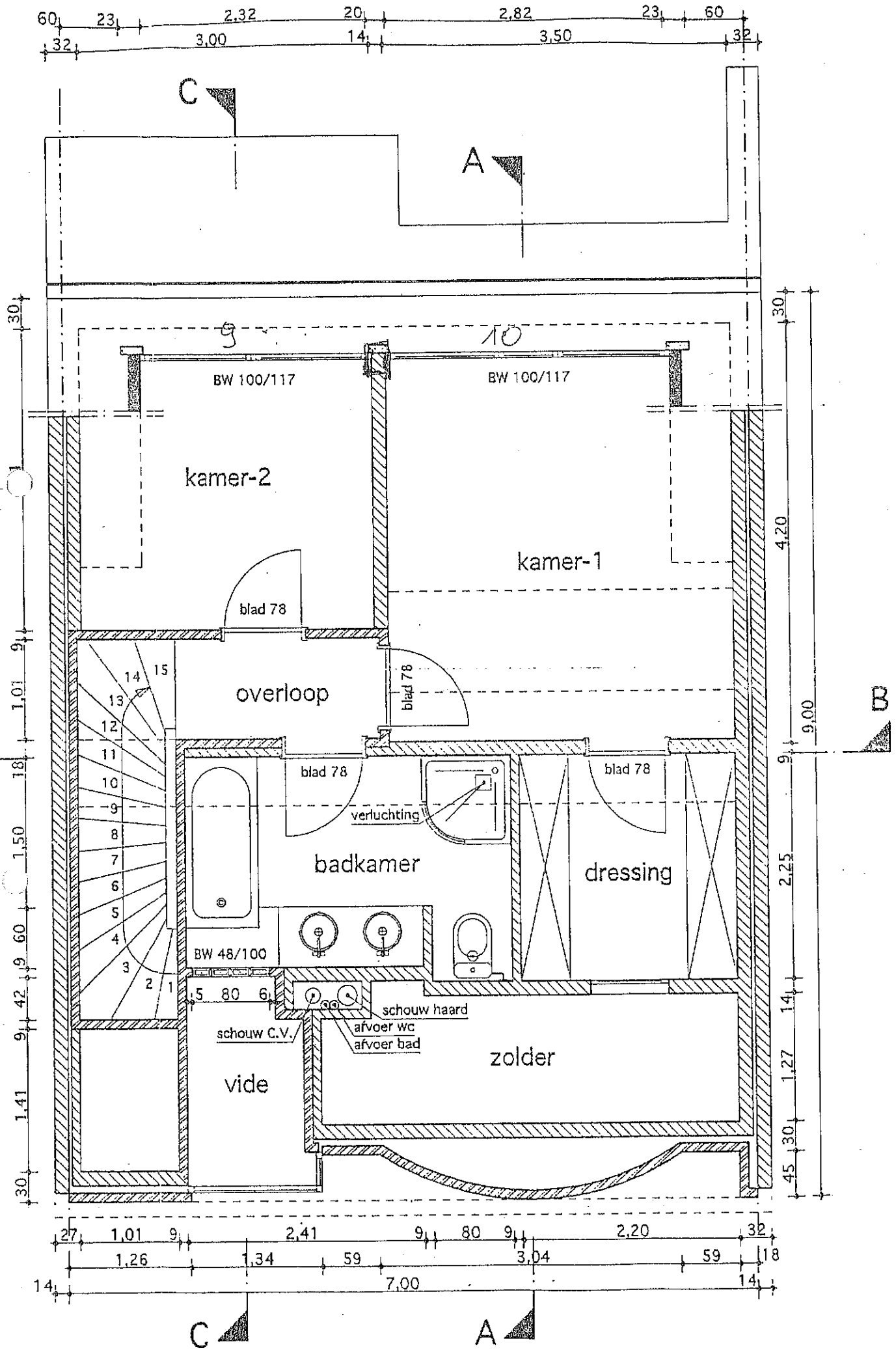
VERDIEPINGSPLAN - 2
