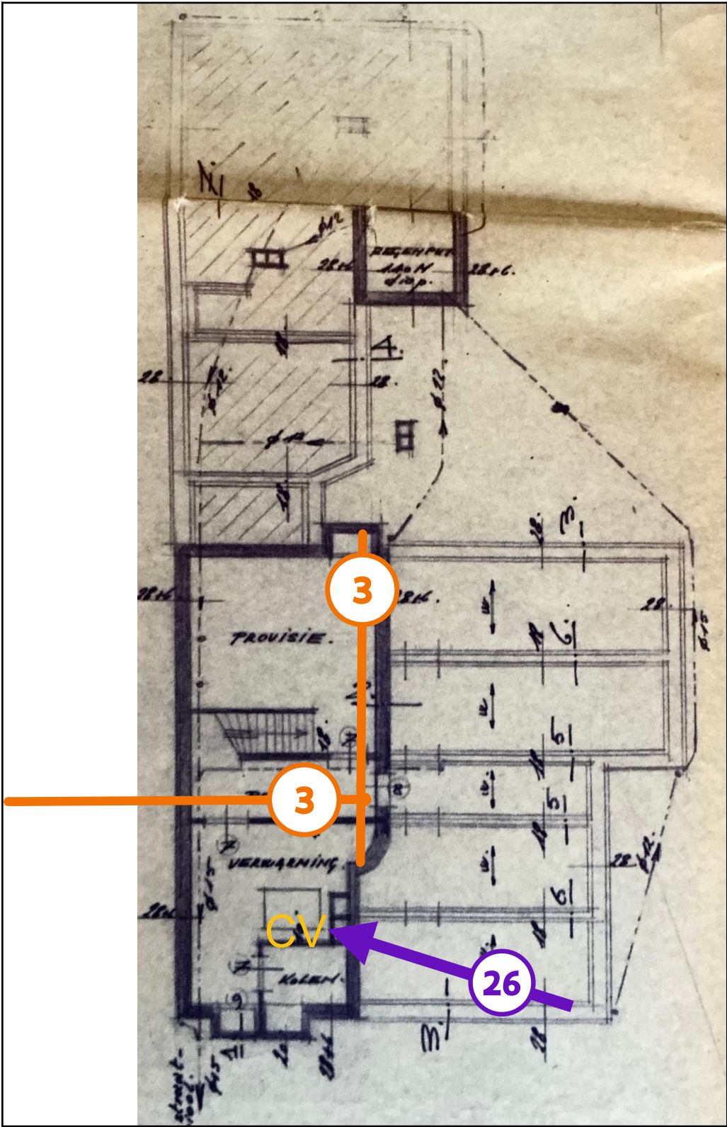
Legende van plan 1.2: kelder
