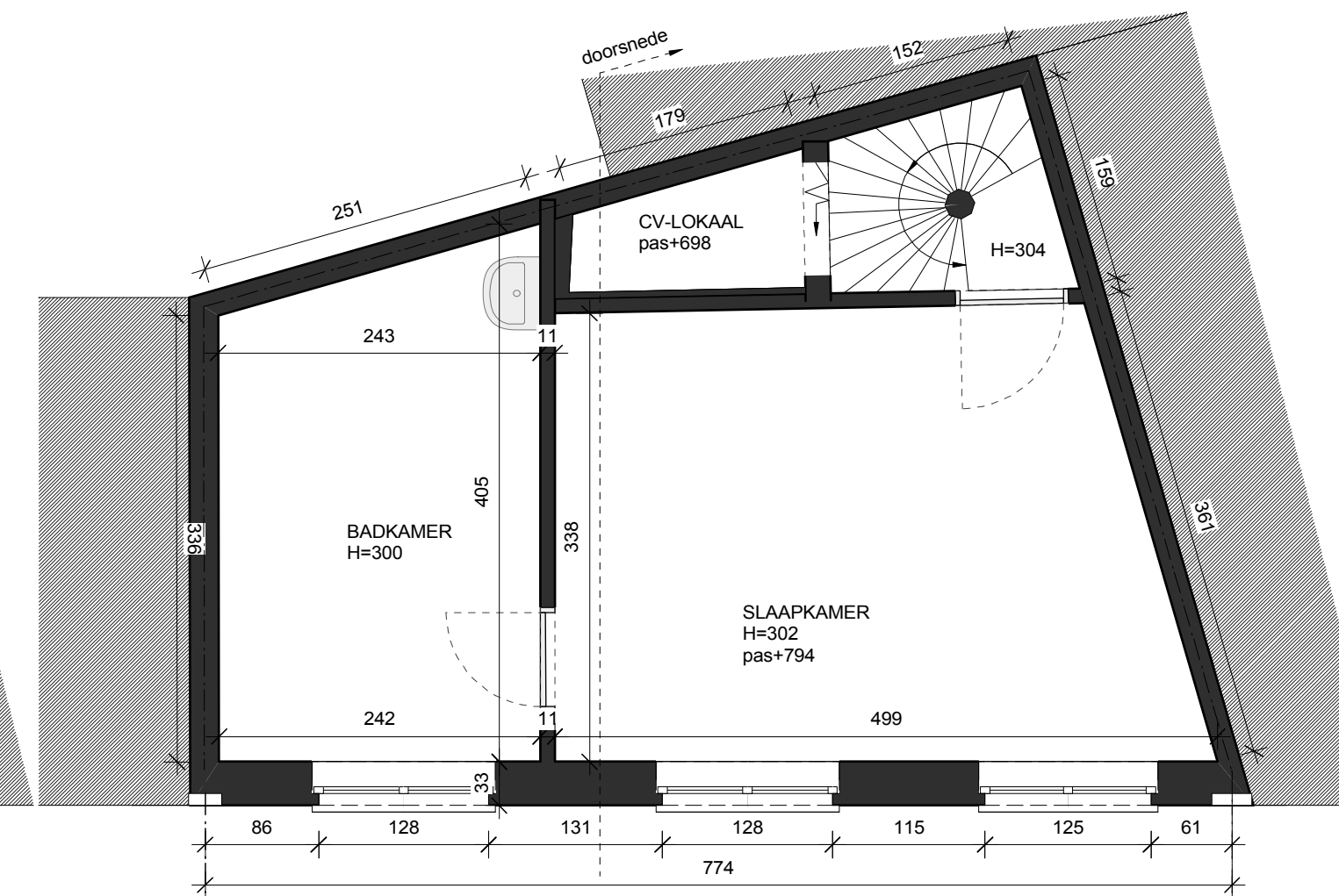
VERDIEP 2 1/50 nieuwe toestand
