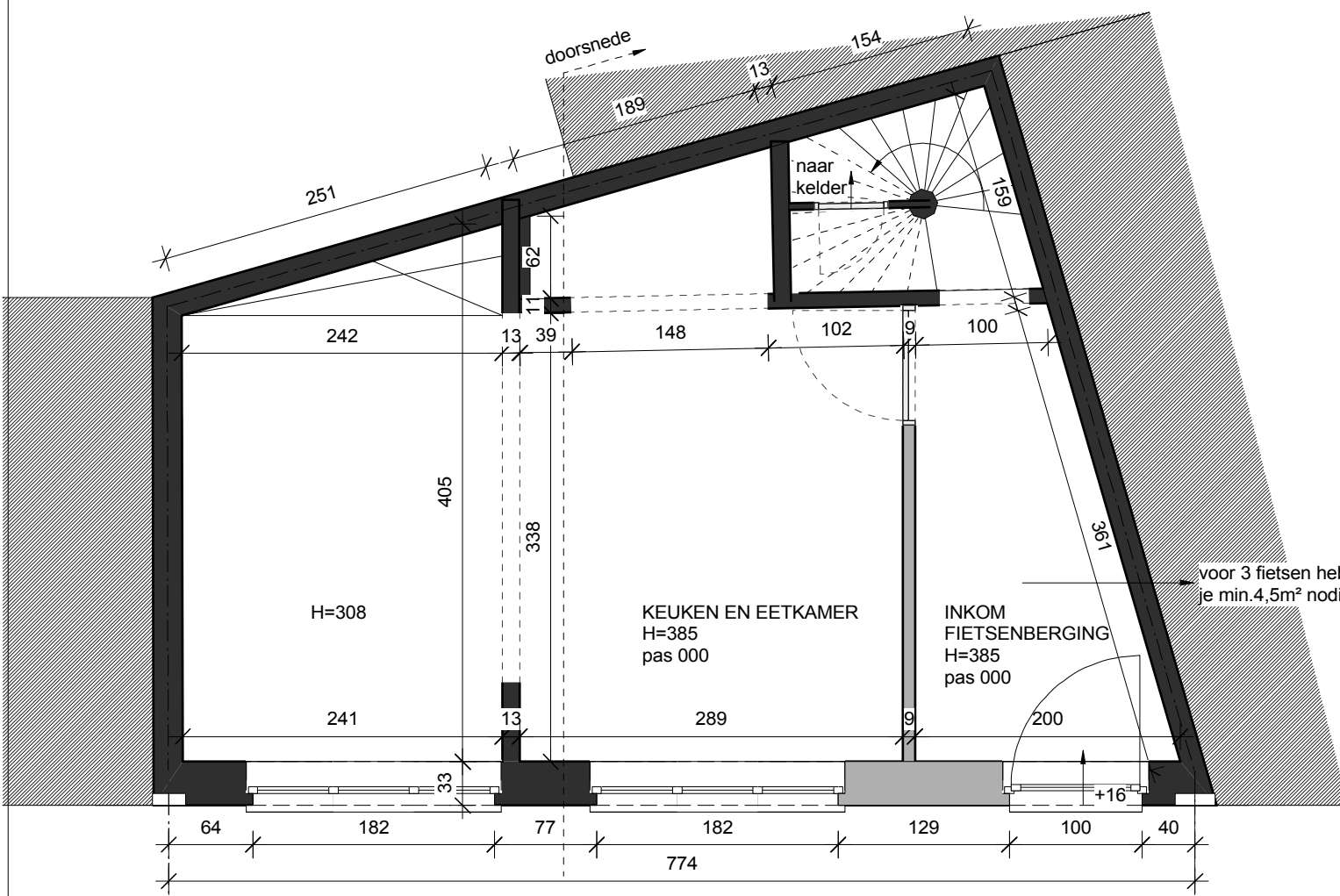
GELIJKVLOERS 1/50 nieuwe toestand
