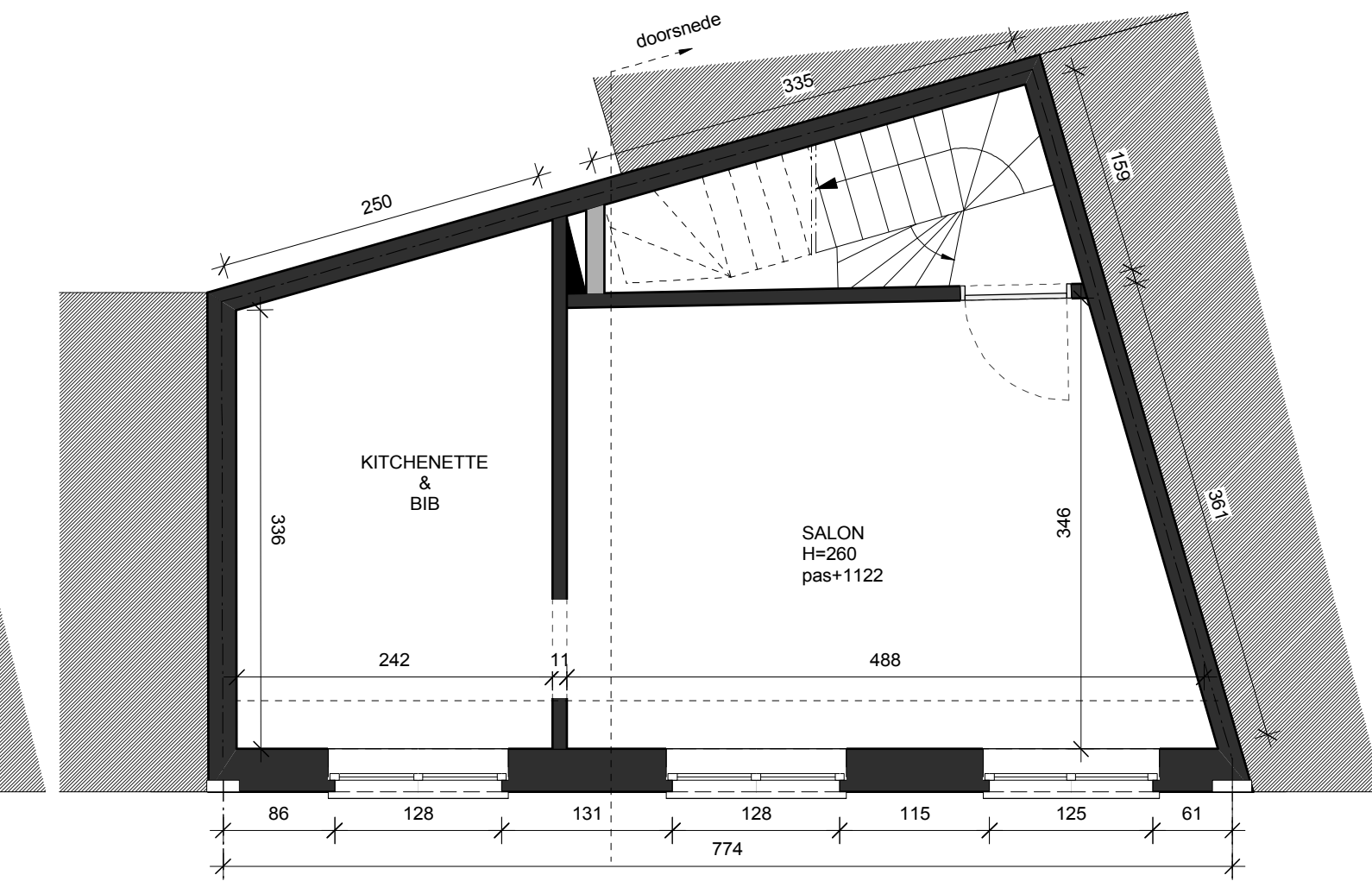
VERDIEP 3 1/50 nieuwe toestand
