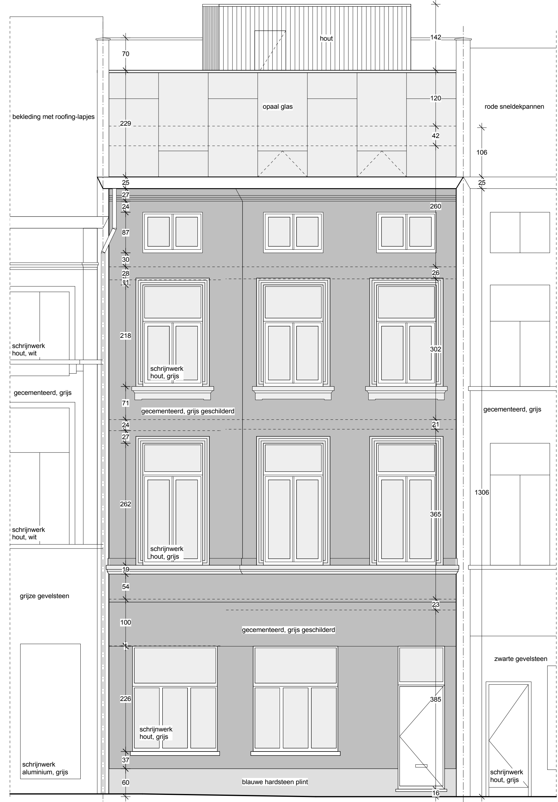
VOORGEVEL 1/50 nieuwe toestand
