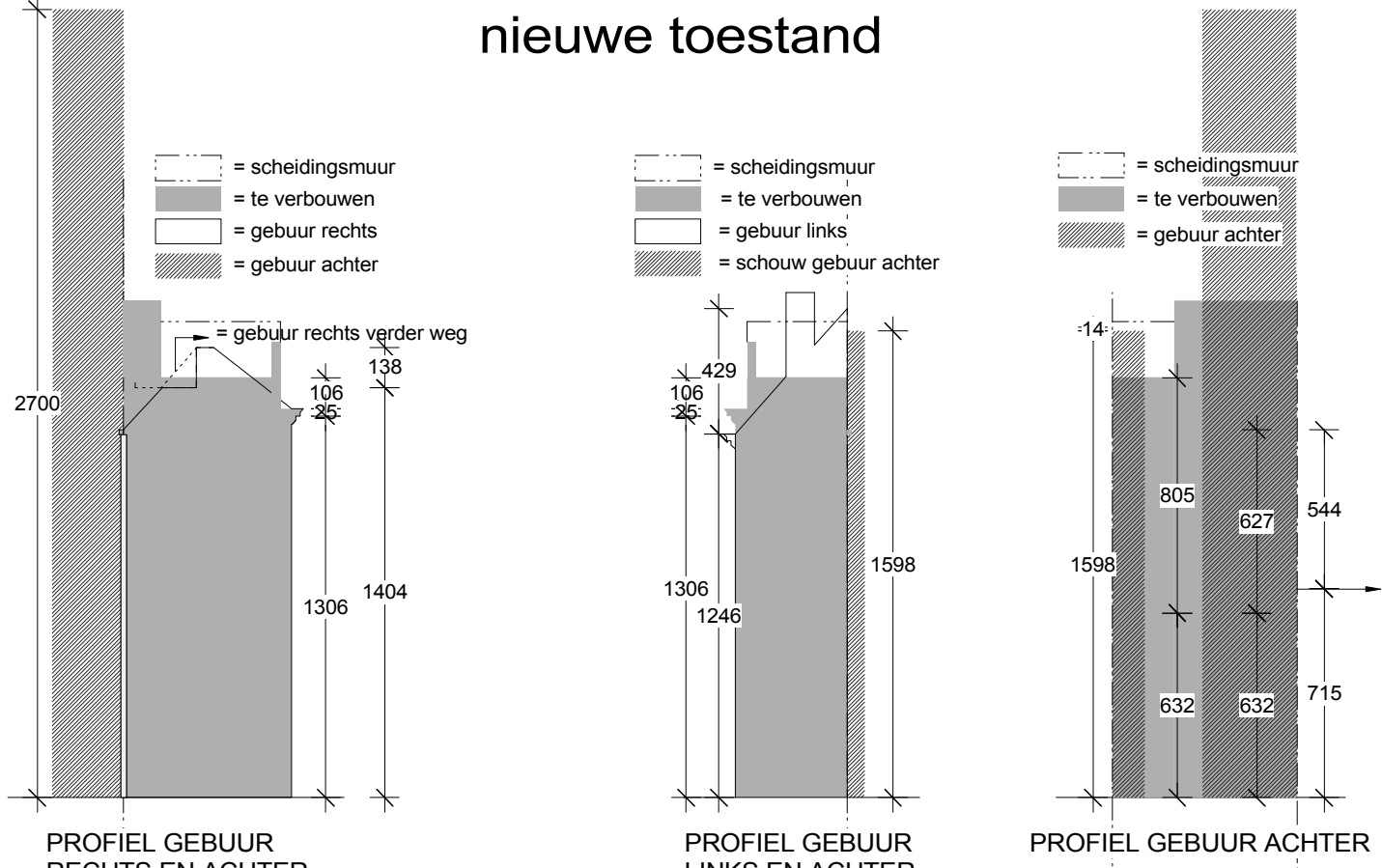
TERREINPROFIEL GEBUREN 1/250 nieuwe toestand
