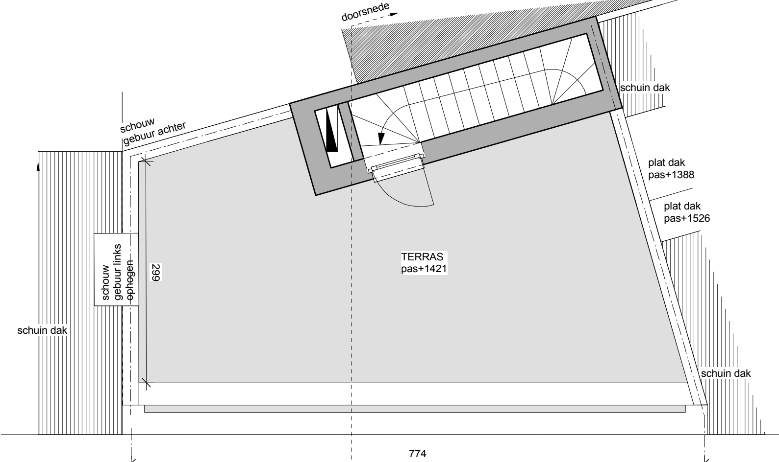
DAKVERDIEP 1/50 nieuwe toestand
