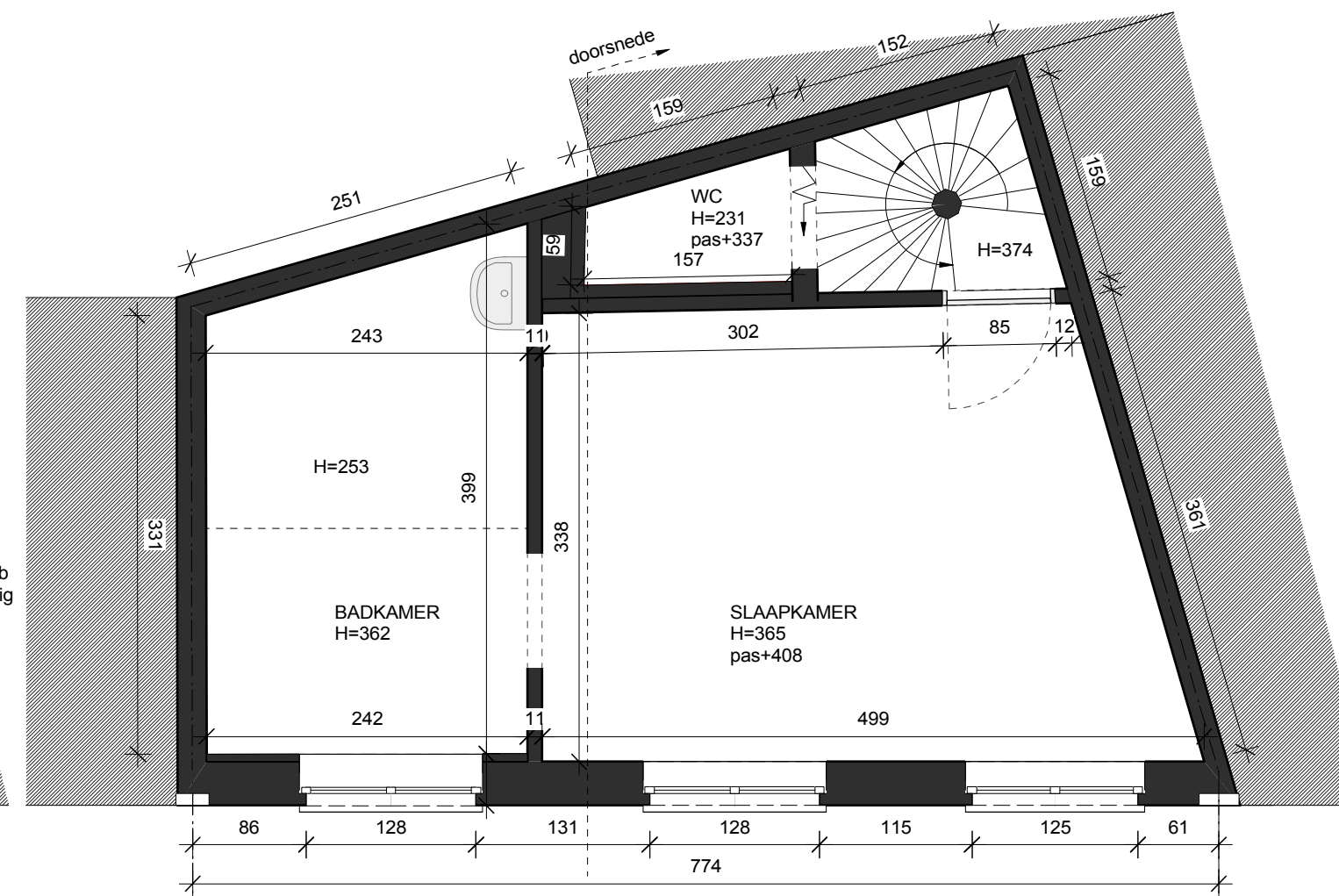
VERDIEP 1 1/50 nieuwe toestand
