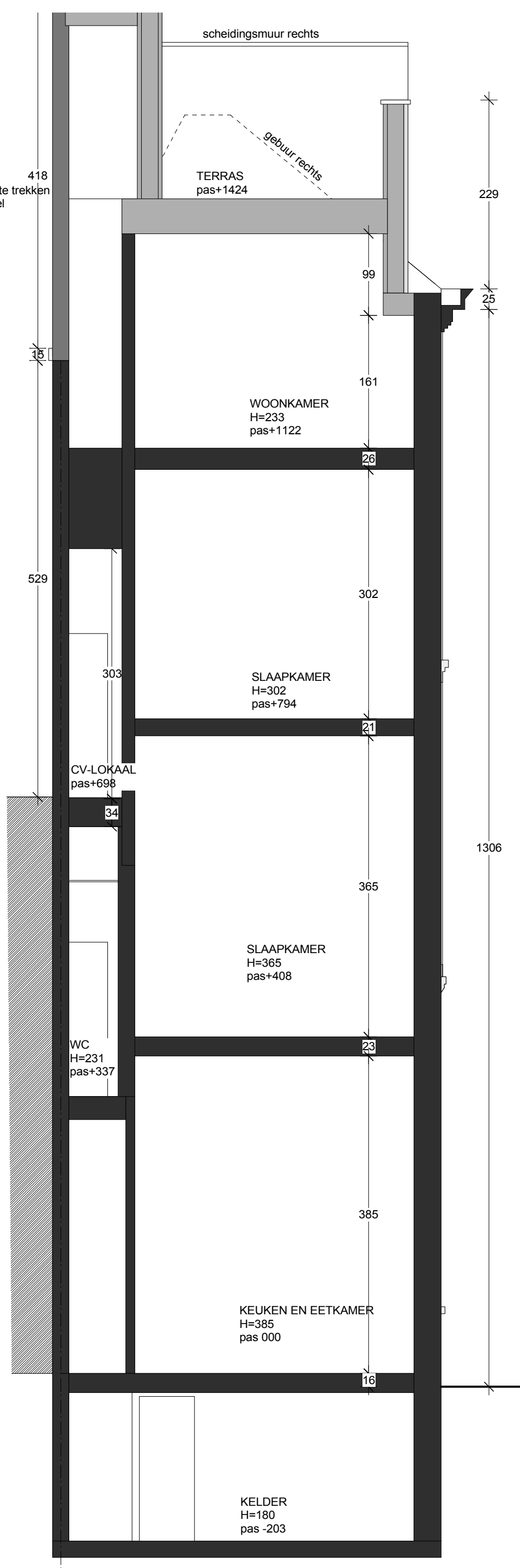
DOORSNEDE 1/50 nieuwe toestand
