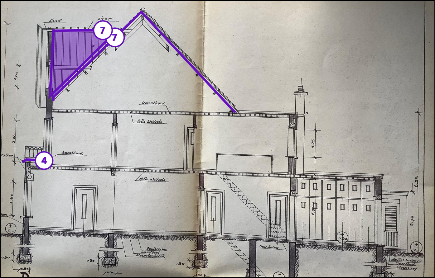
Legende van plan 1.7: Doorsnede
