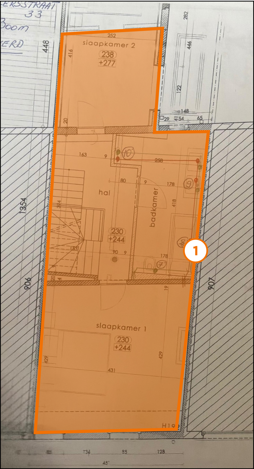
Legende van plan 1.6: Eerste verdiep plafond
