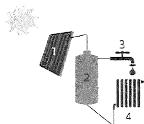
1. Zonnecollector | 2. Opslagvat zonnecollector | 3. Sanitair warm water | 4. Afgifteenheid voor ruimteverwarming (radiator)
