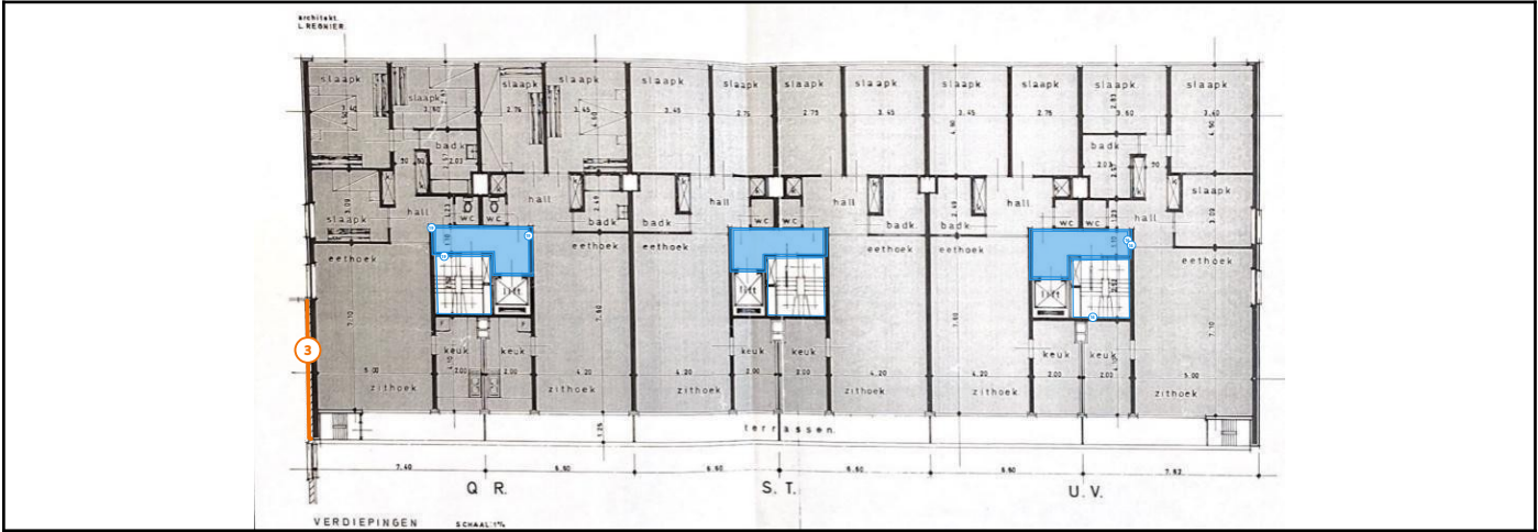
Legende van plan 1.11: Verdieping +7
