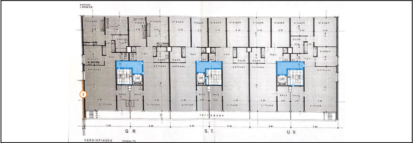
Legende van plan 1.17: Verdieping +13
