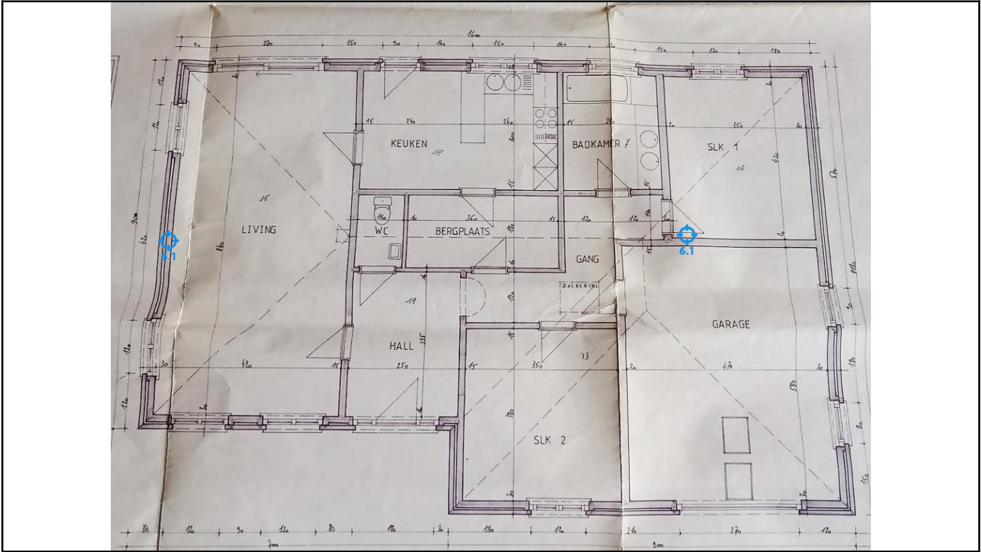
Legende van plan 1.6: Gelijkvloers plan
