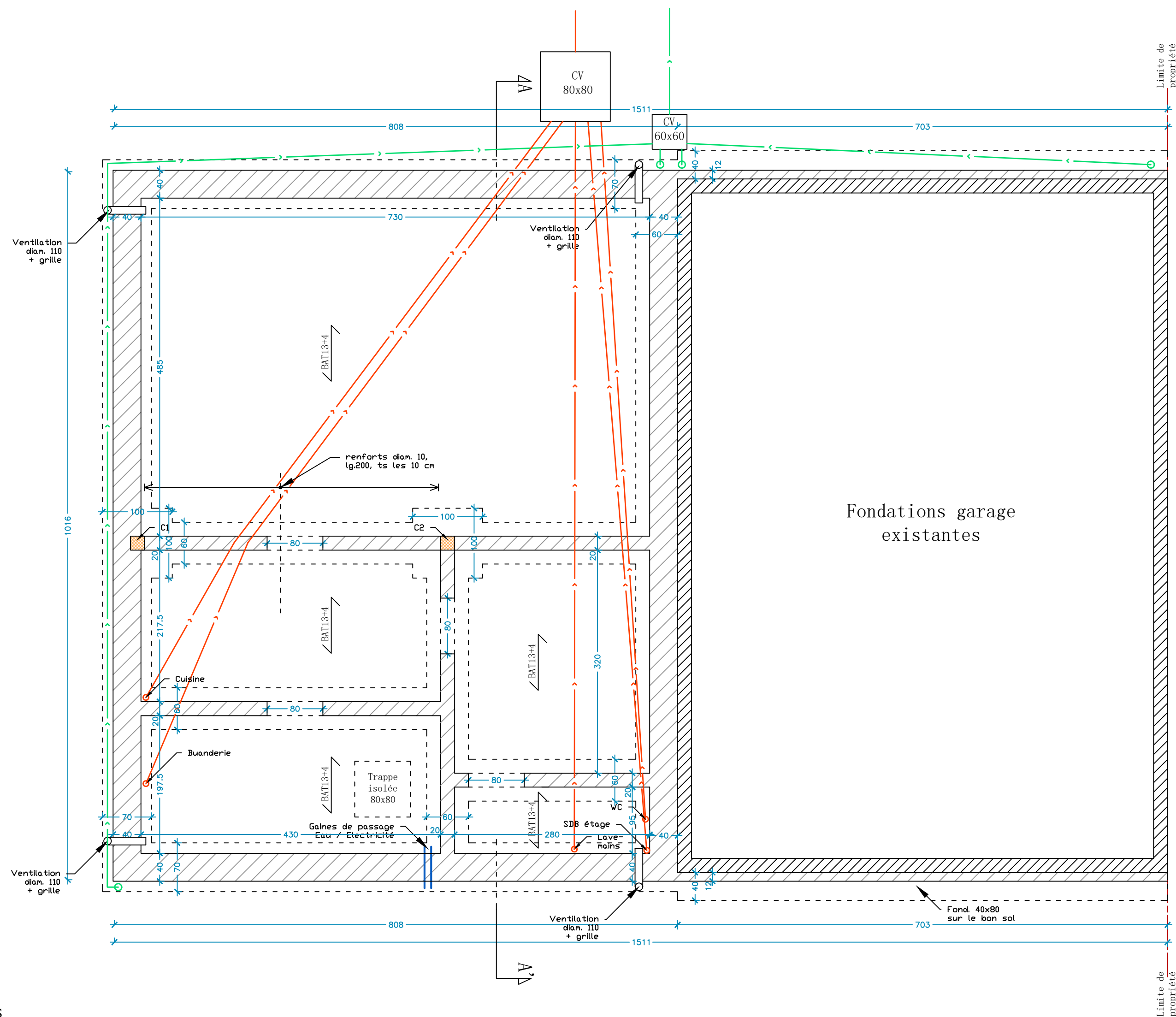
Vue en plan - Fondations
