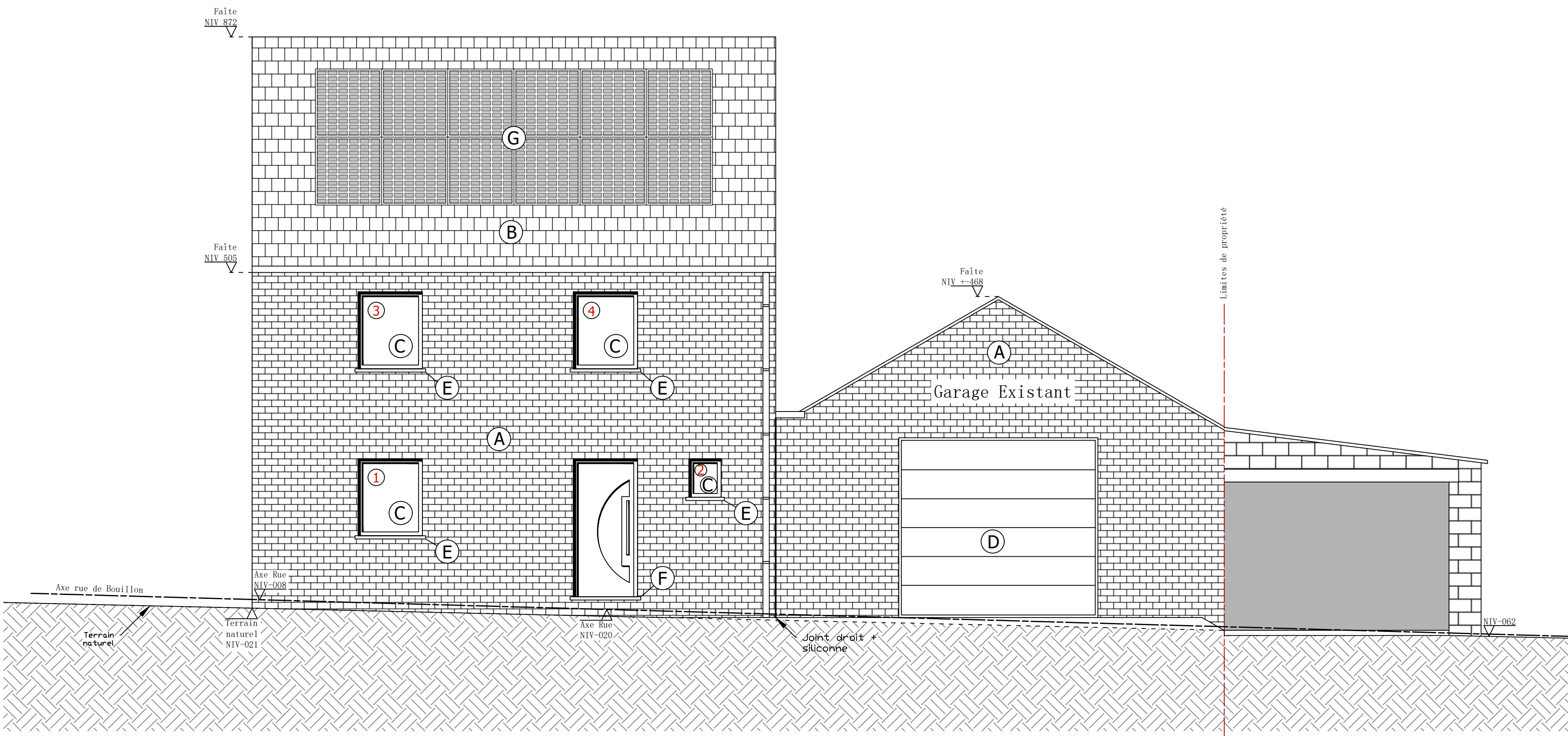
Façade avant (Est)
