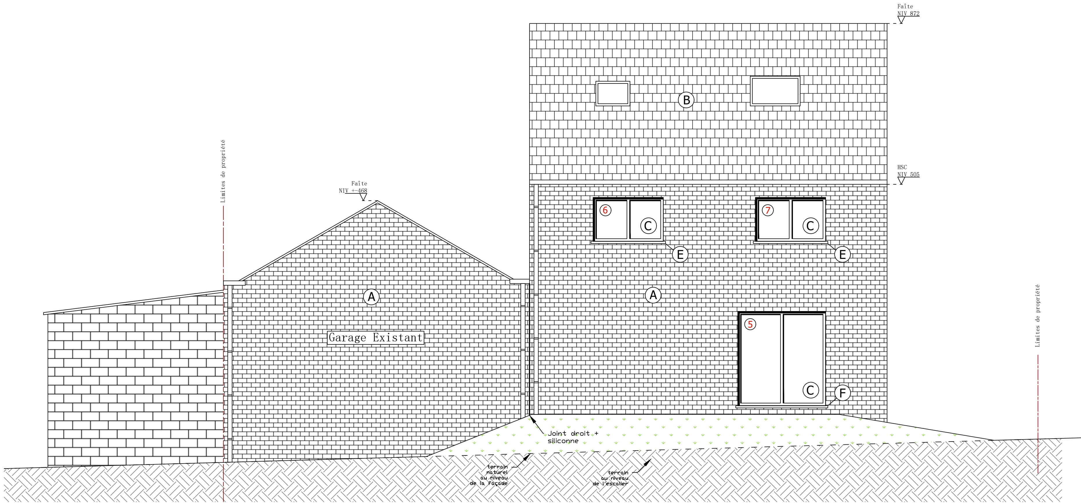
Façade arrière (Ouest)
