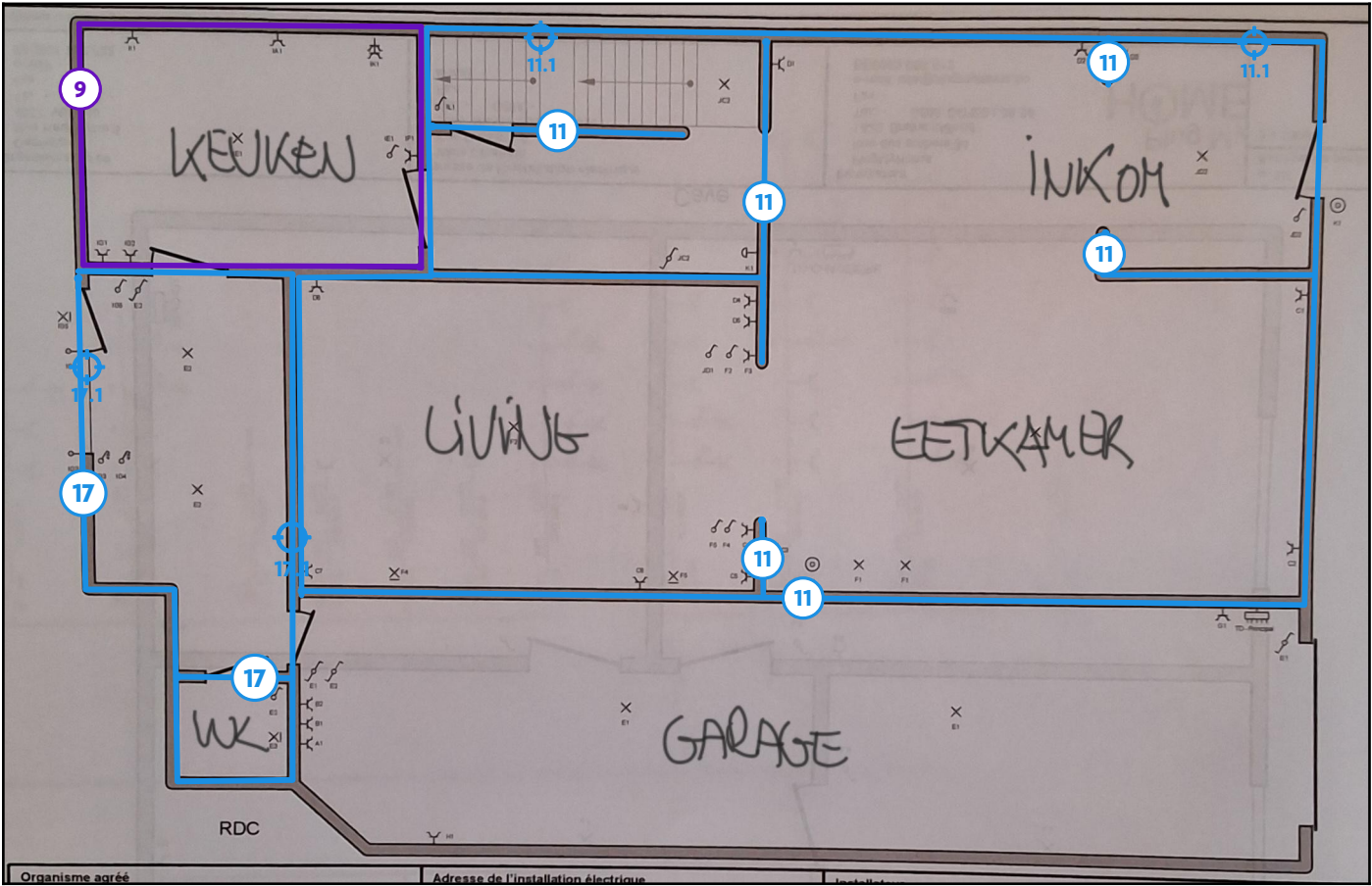
Legende van plan 1.4: Gelijkvloers (wanden)
