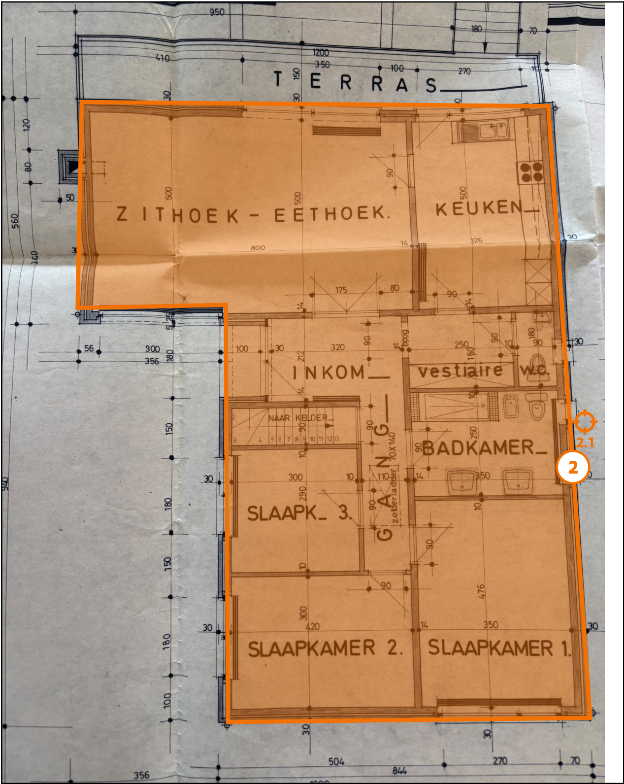
Legende van plan 1.3: Plan - Gelijkvloers
