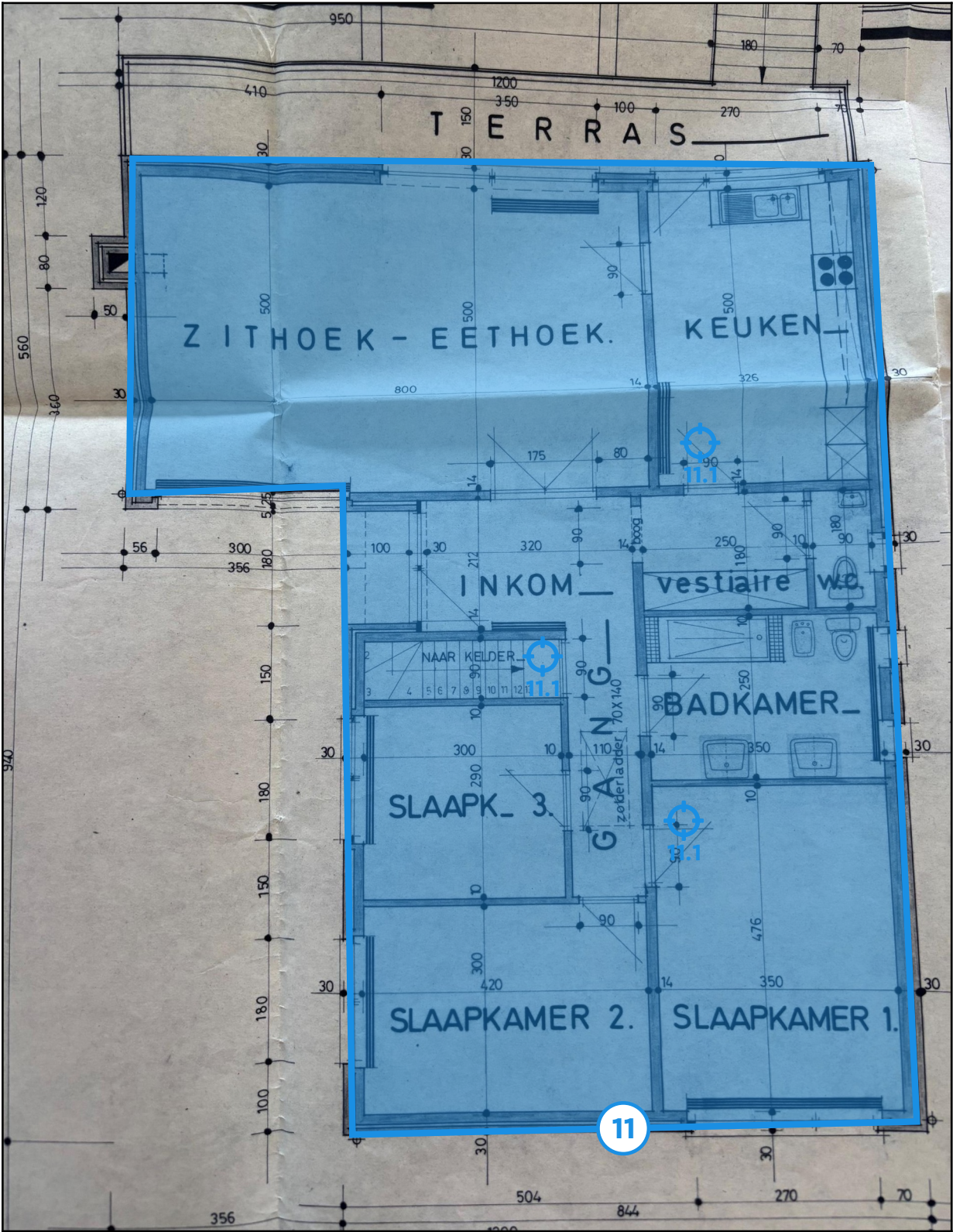
Legende van plan 1.2: Plan - Gelijkvloers
