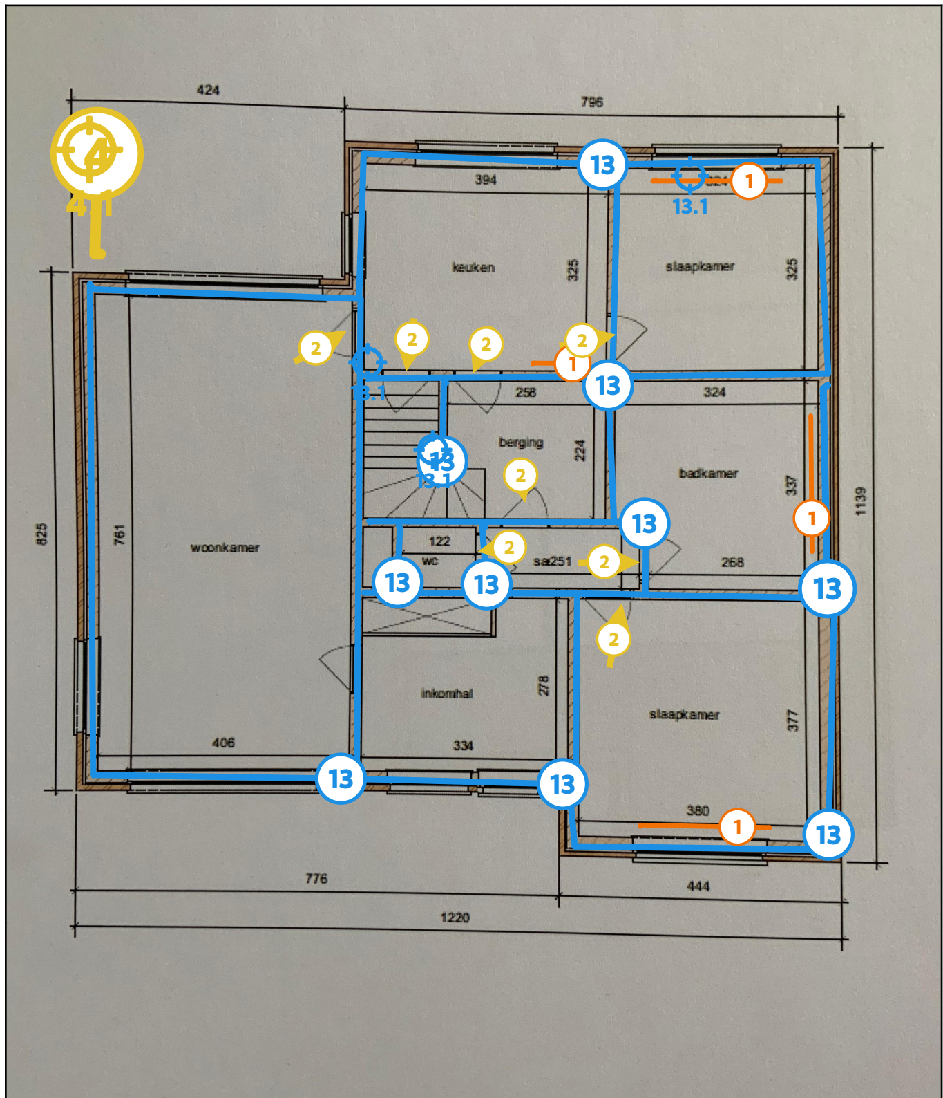
Legende van plan 1.3: Grondplan glv
