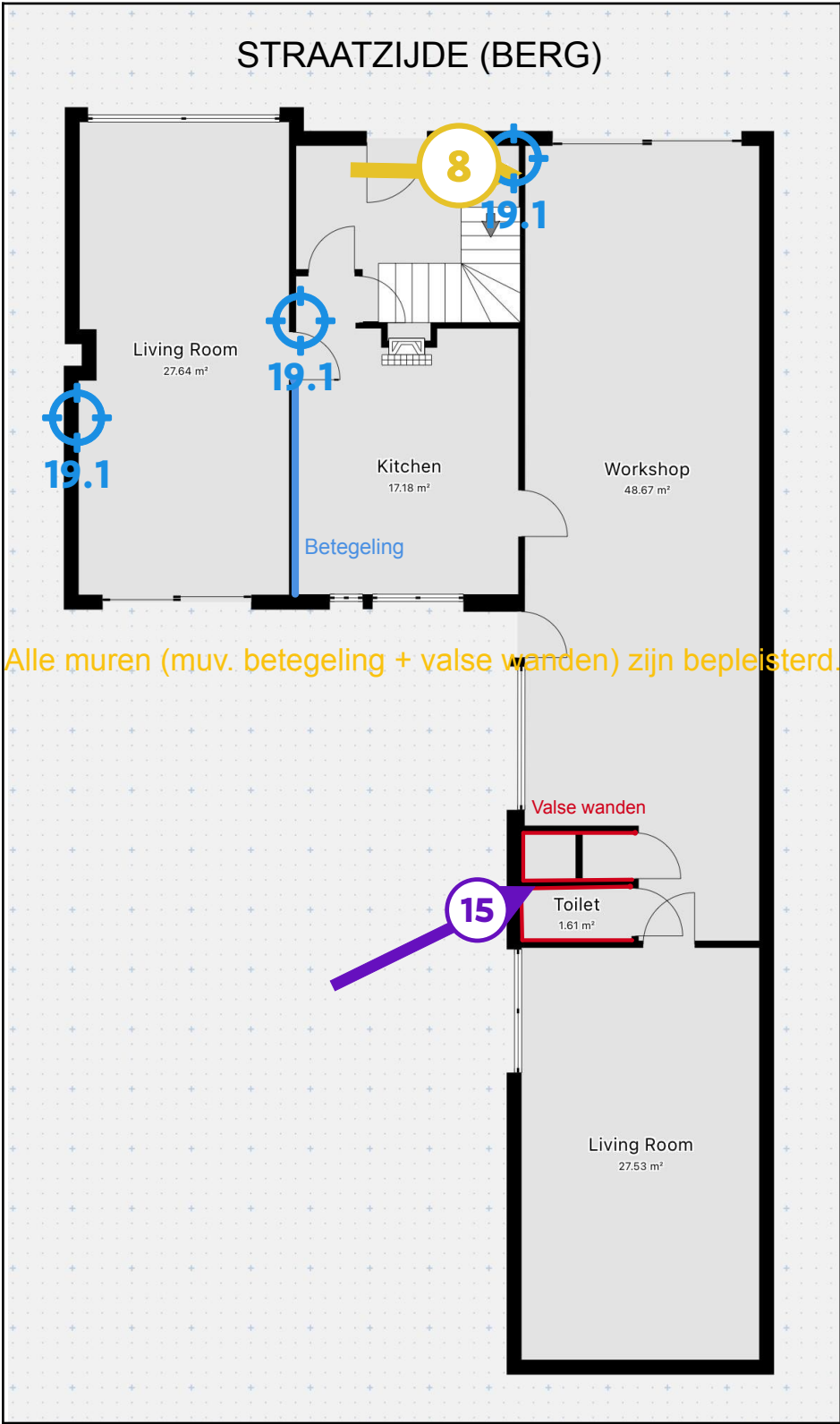
Legende van plan 1.3: Grondplan woning/winkel GLV
