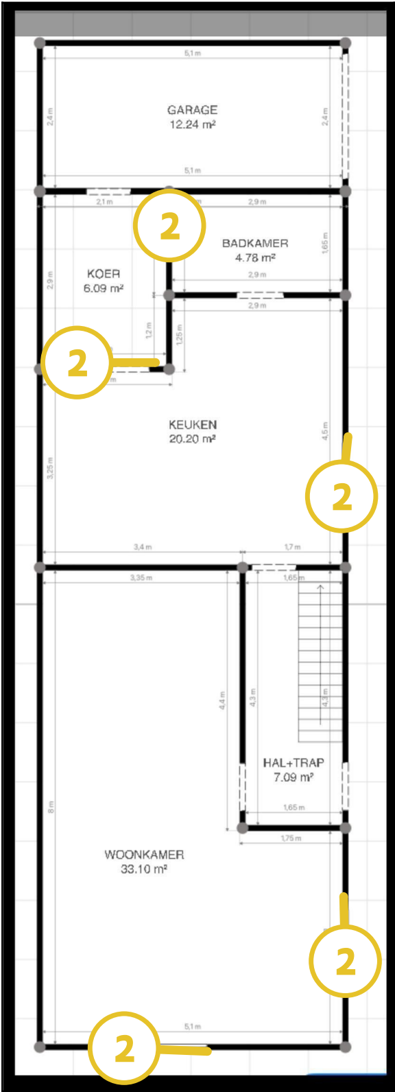
Legende van plan 1.6: Gelijkvloers woning
