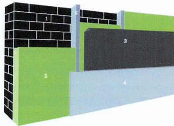
1. Buitenmuur | 2. Isolatie | 3. Vochtsscherf | 4. Afwerkingslaag | 5. Stijl- en regelwerk (optioneel)
