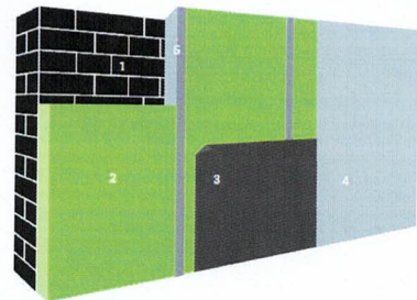
1. Buitengevel | 2. Isolatie | 3. Dampsscherf | 4. Binnenafwerking | 5. Stijl- en regelwerk (optioneel)
