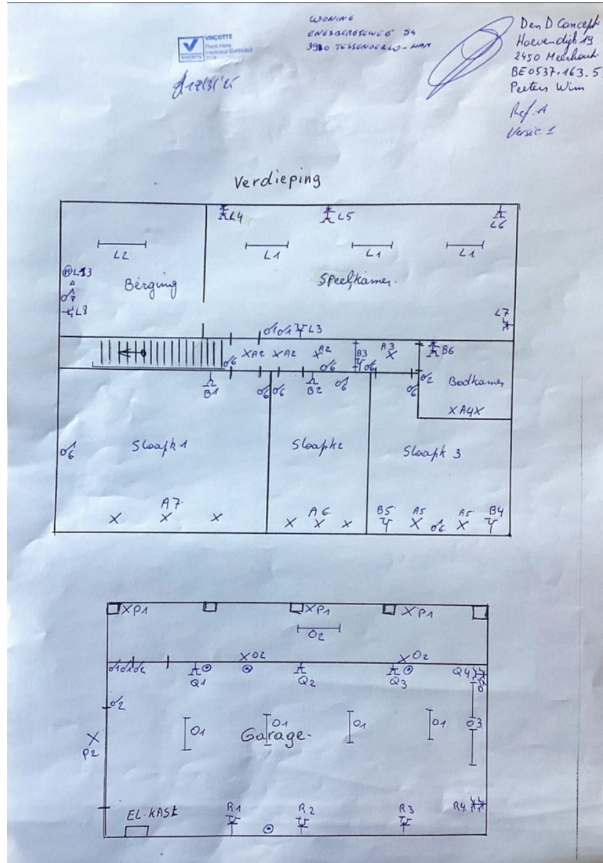
( Situatieplannen )
