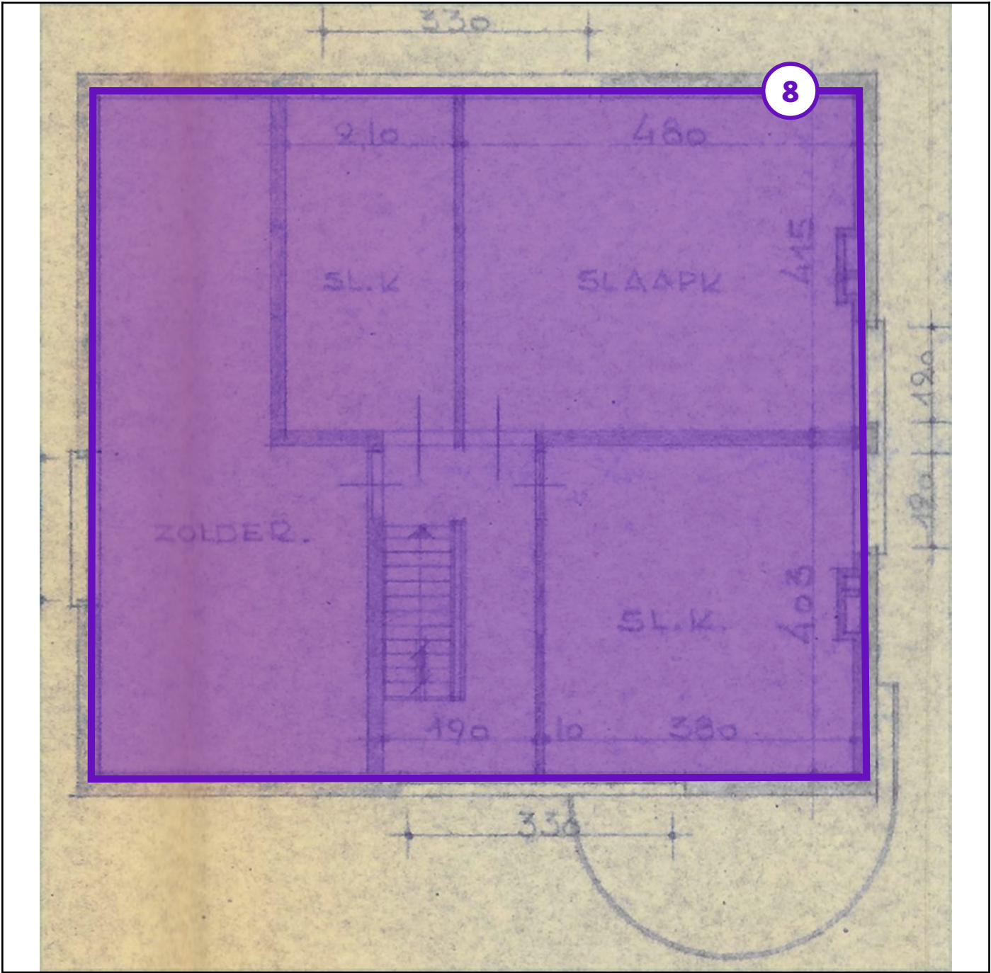
Legende van plan 1.13: Plan woning eerste verdieping 6
