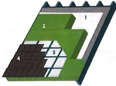
1. Damperscherm | 2. Isolatie | 3. Onderdak | 4. Dakbedekking
