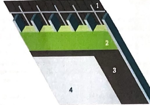
1. Onderdak | 2. Isolatie | 3. Damperscherm | 4. binnenafwerking
