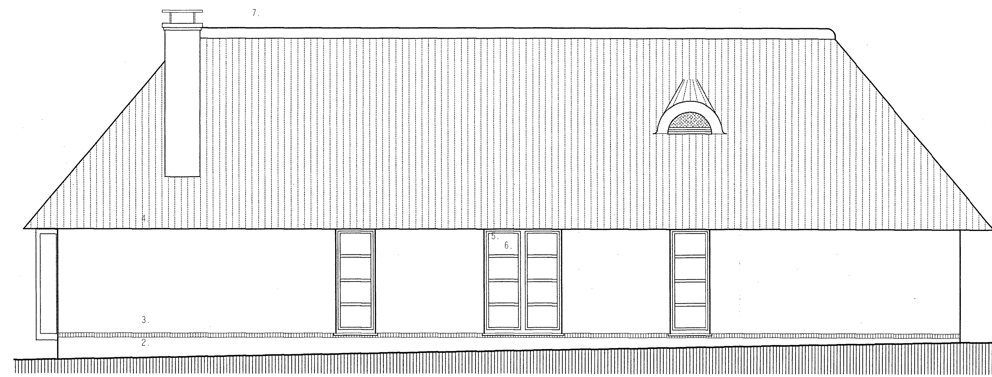
LINKERGEVEL
