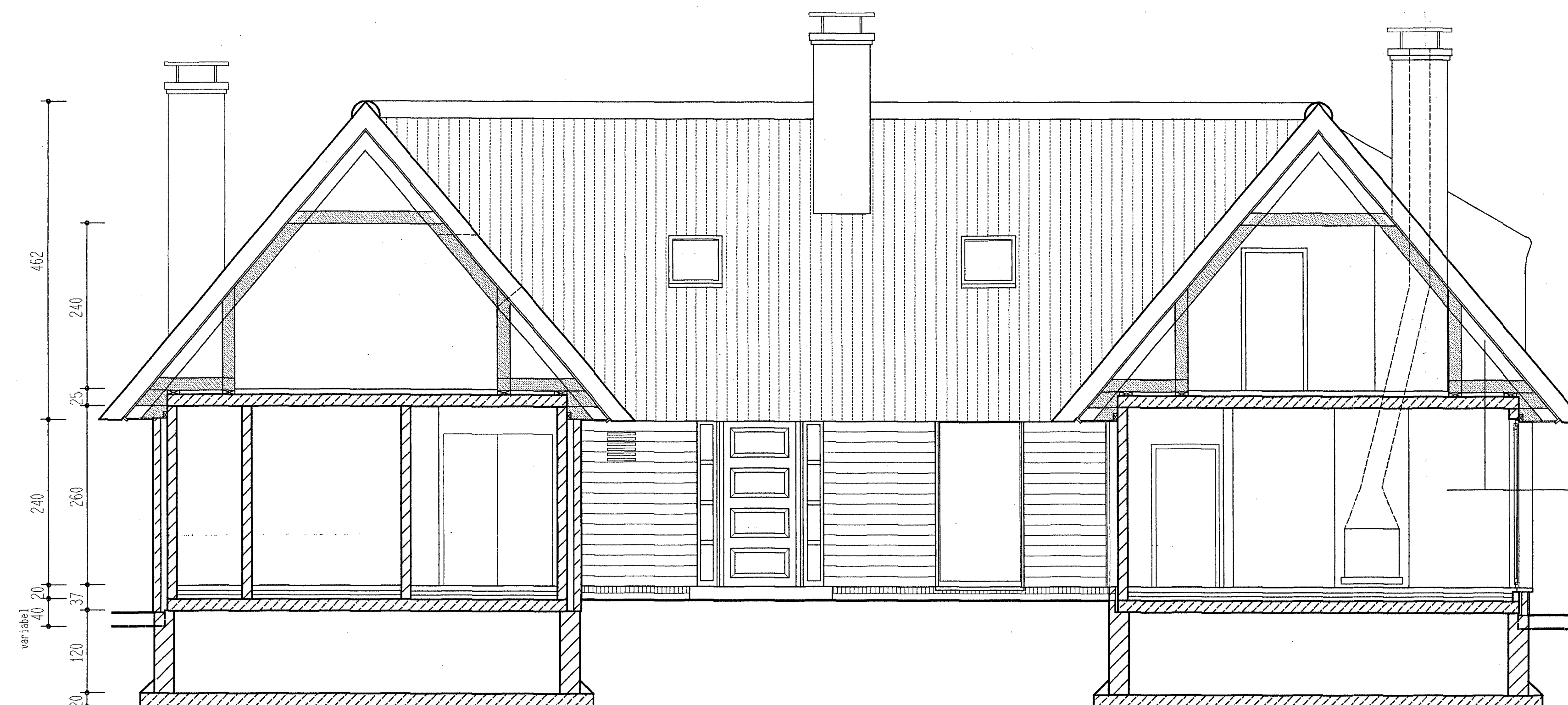
DOORSNEDE AA
