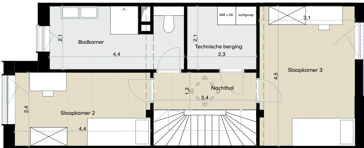
niv +2
