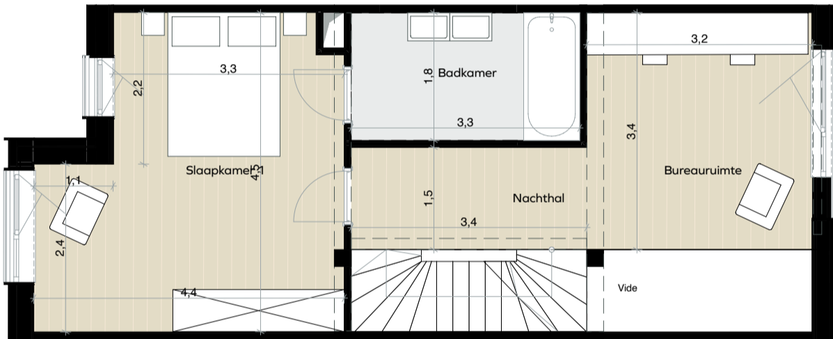
niv +1
