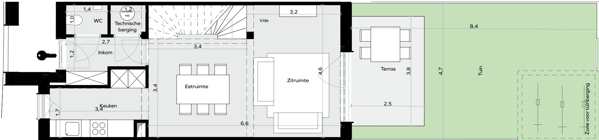
gelijkvloers
