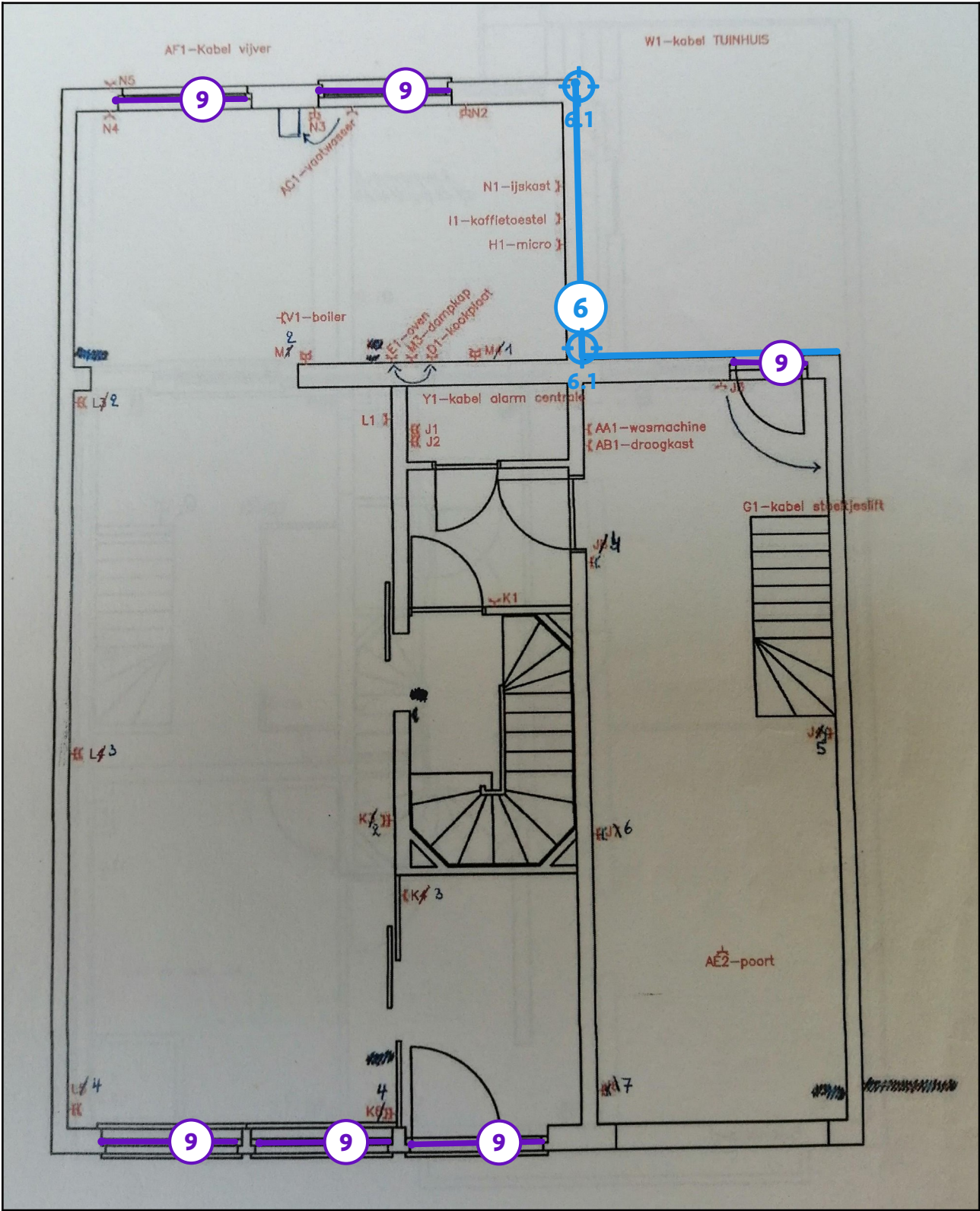
Legende van plan 1.1: grondplan gelijkvloers
