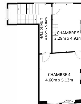
2EME ETAGE
