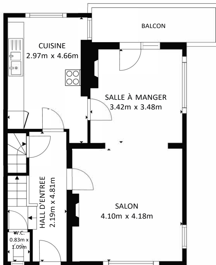
REZ-DE-CHAUSSEE
