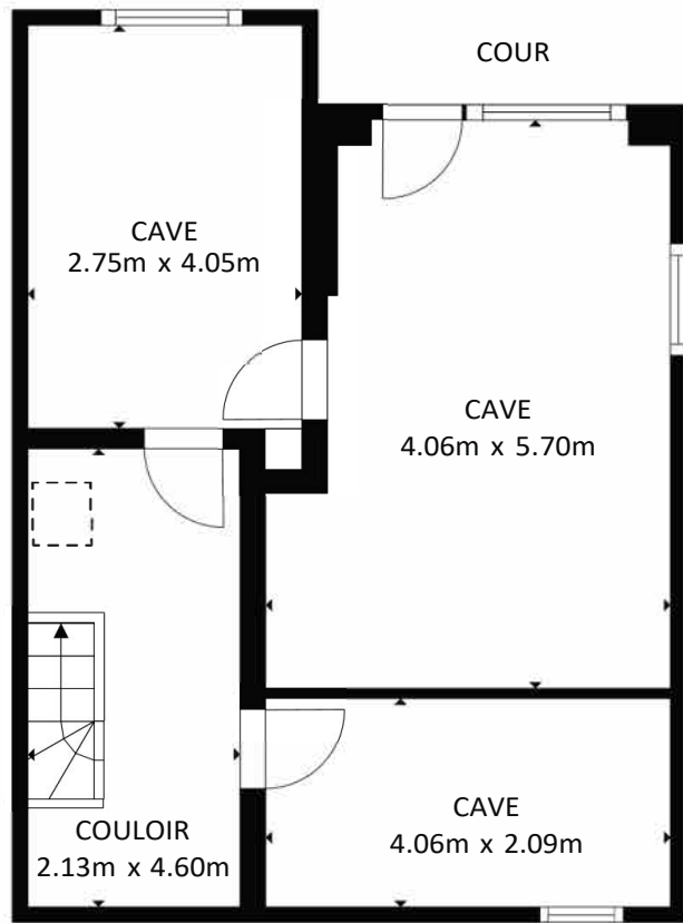
SOUS-SOL
