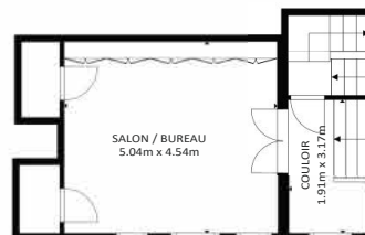
ENTRESOL
