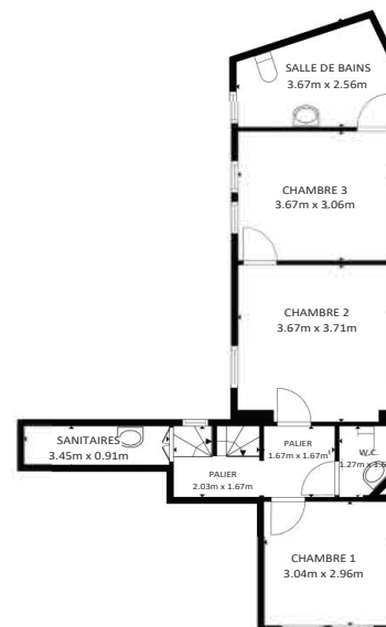
1ER ETAGE
