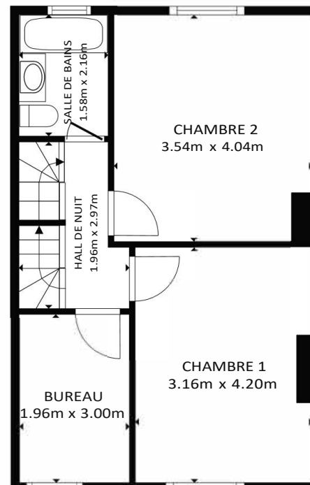
1ER ETAGE
