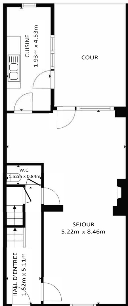
REZ-DE-CHAUSSEE
