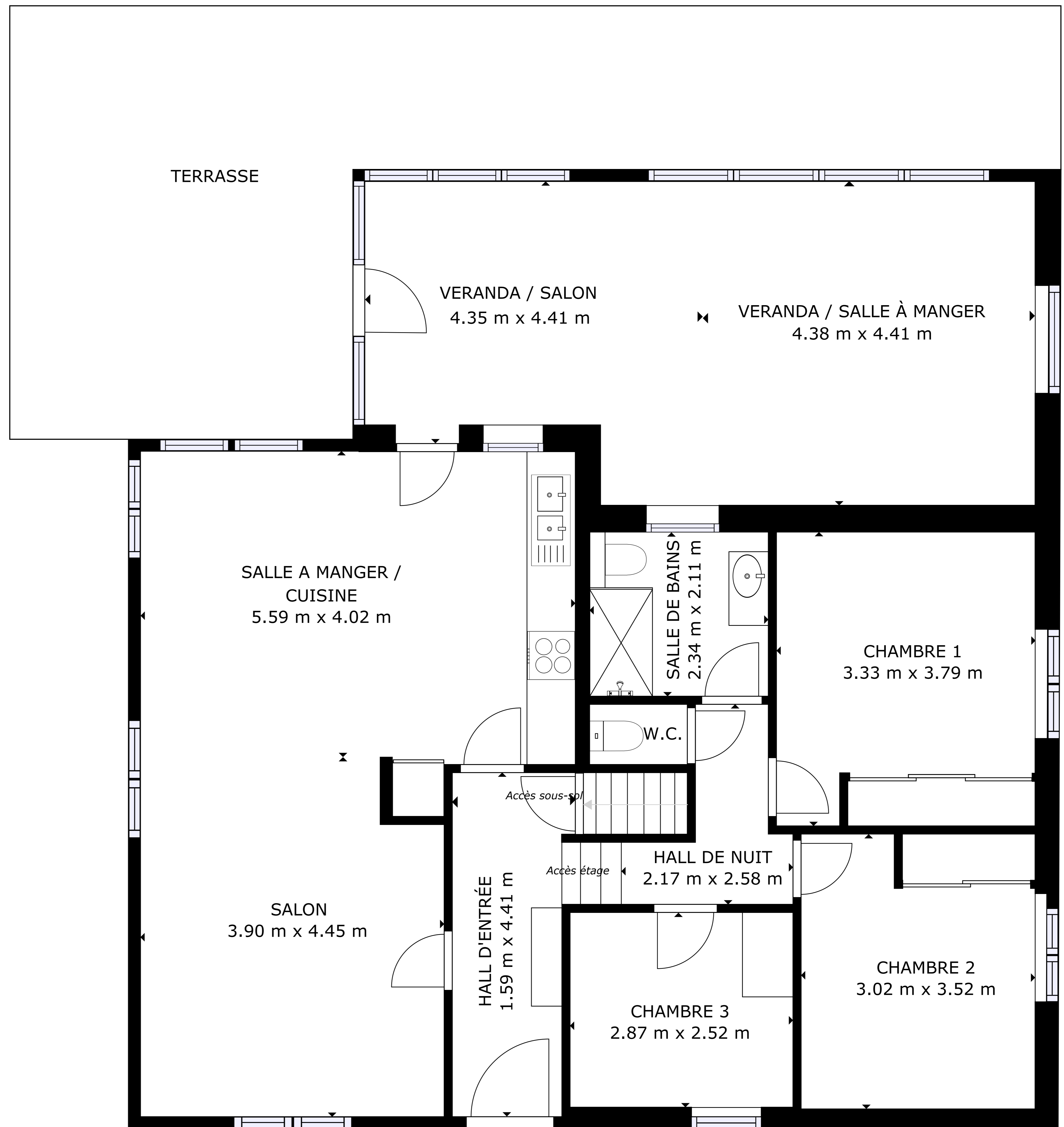
REZ / ETAGE
