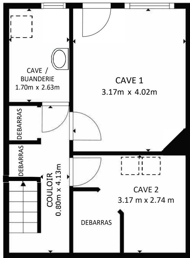
SOUS-SOL
