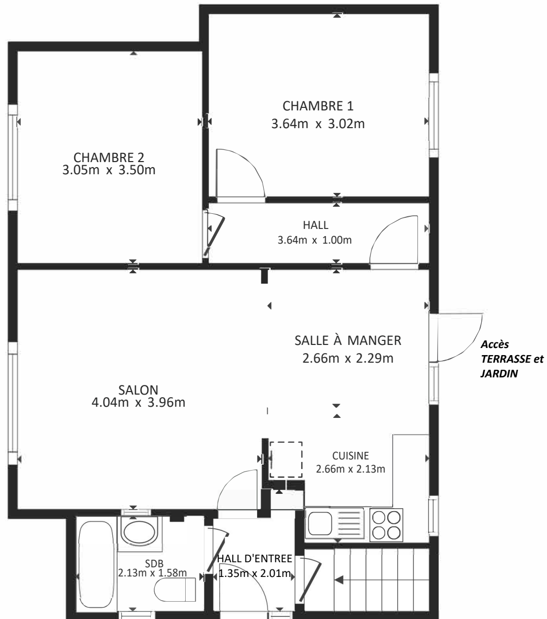
REZ-DE-CHAUSSEE
