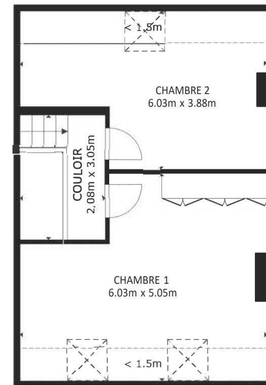
2EME ETAGE
