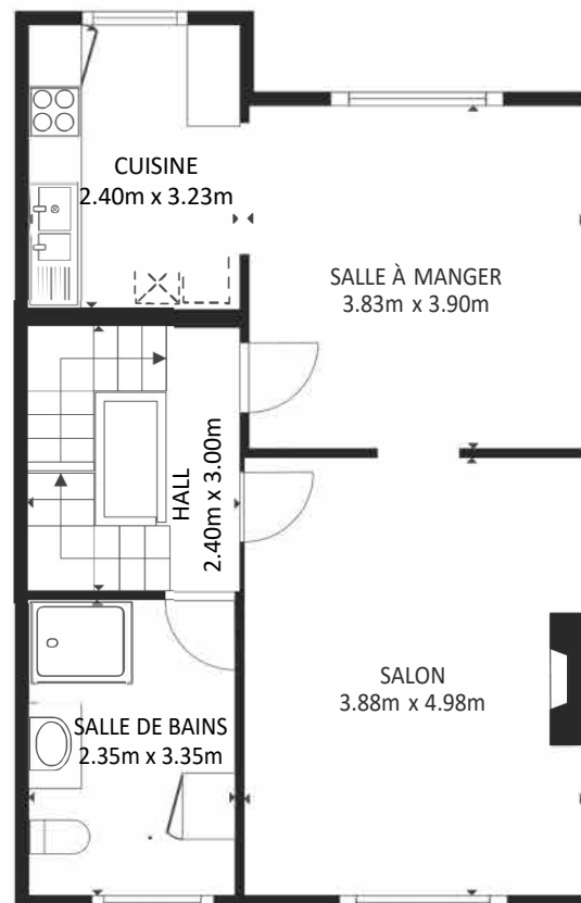
1ER ETAGE
