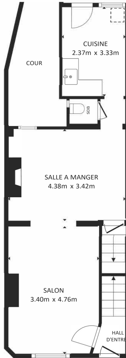
REZ-DE-CHAUSSEE
