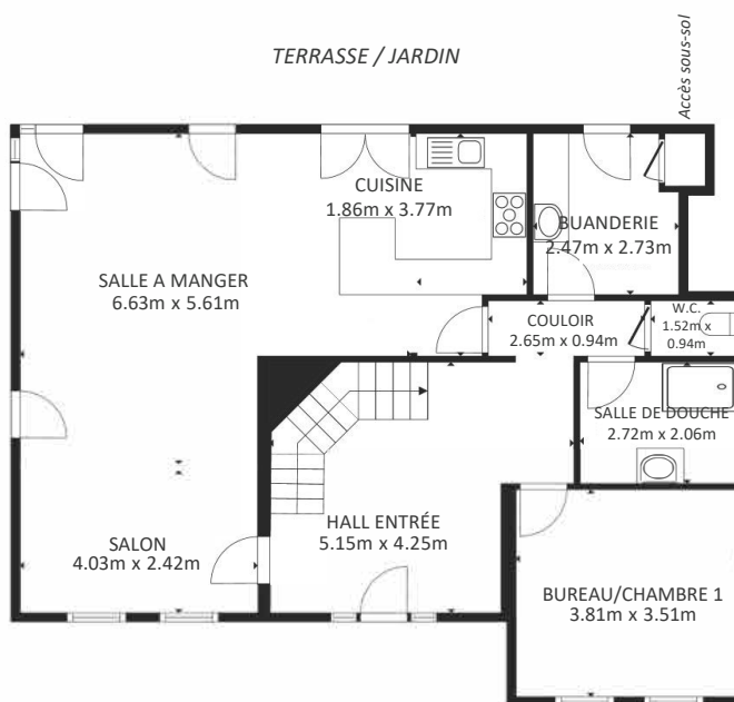
REZ-DE-CHAUSSEE
