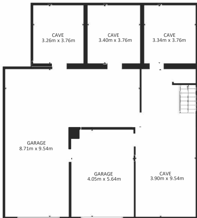
SOUS-SOL
