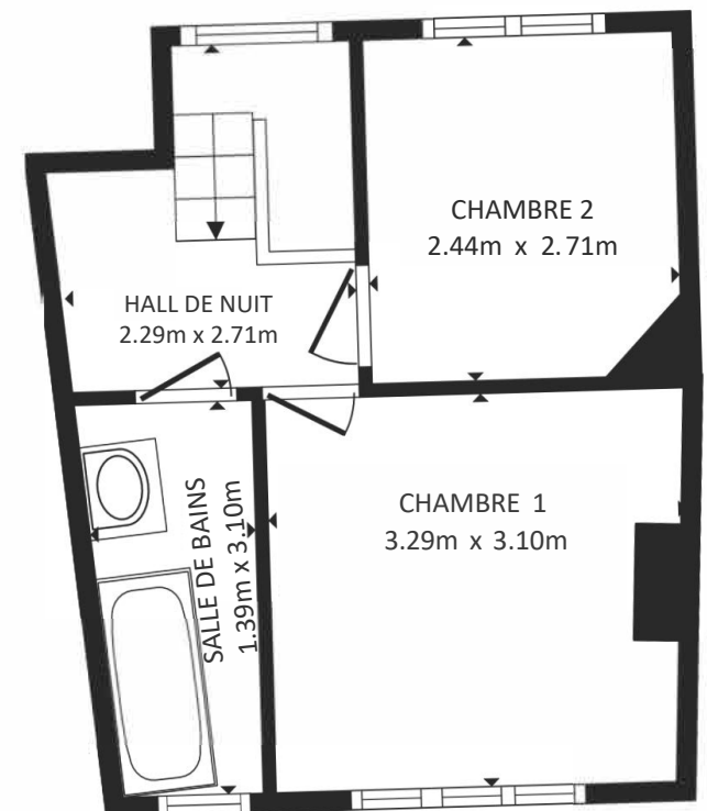
1ER ETAGE
