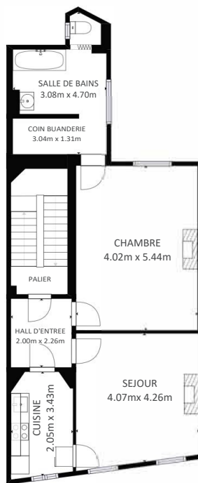
1ER ETAGE
