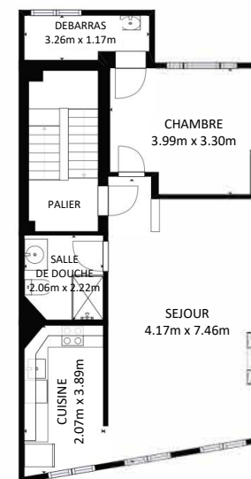
3EME ETAGE
