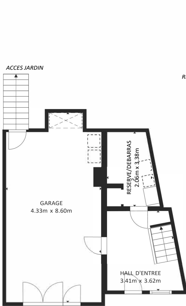
REZ-DE-CHAUSSEE
