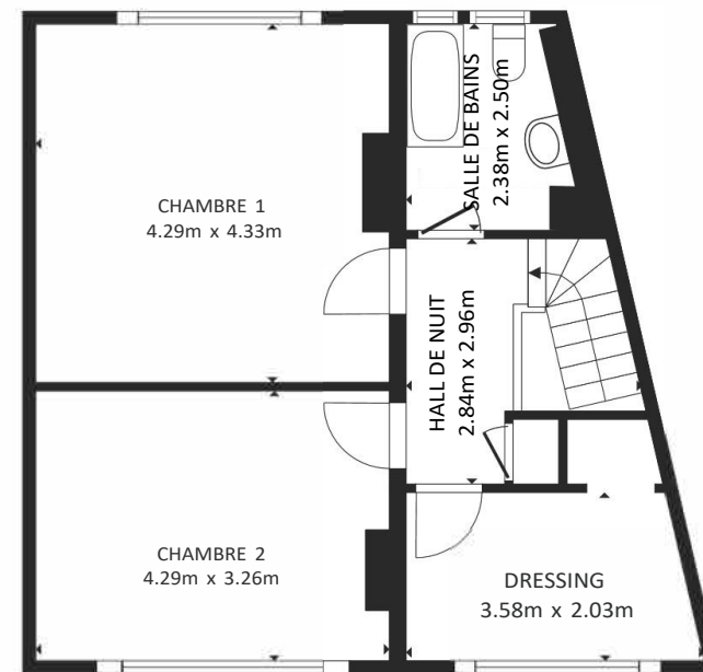
2EME ETAGE
