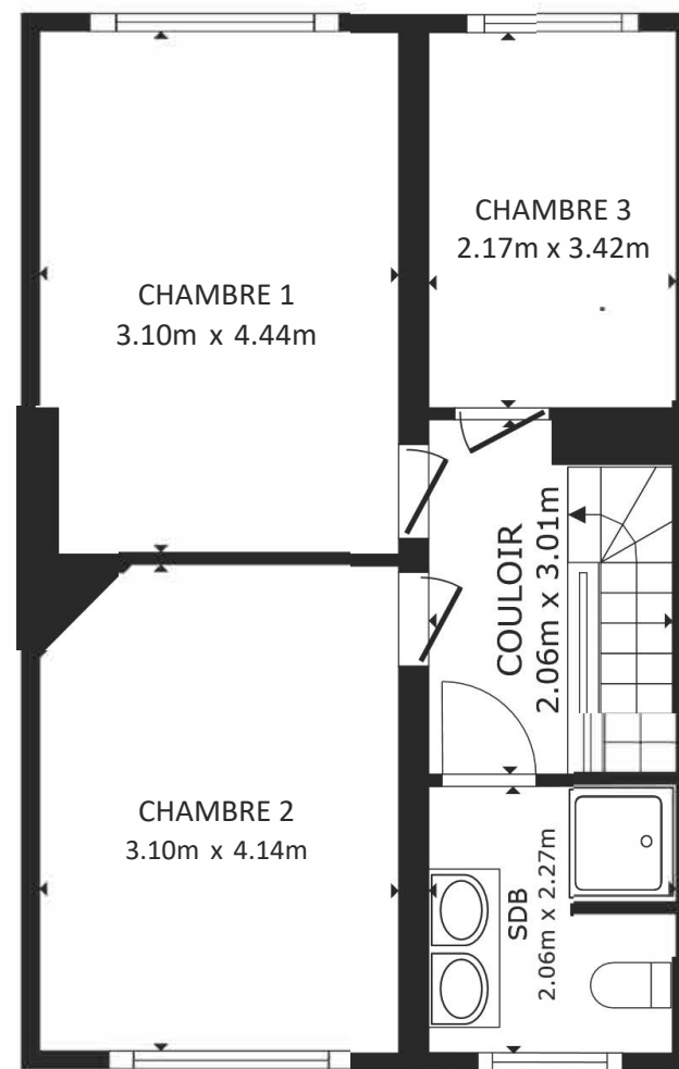
1ER ETAGE
