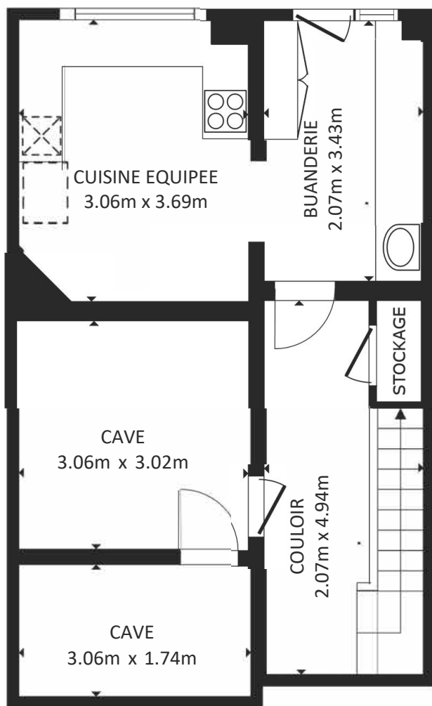
SOUS-SOL
