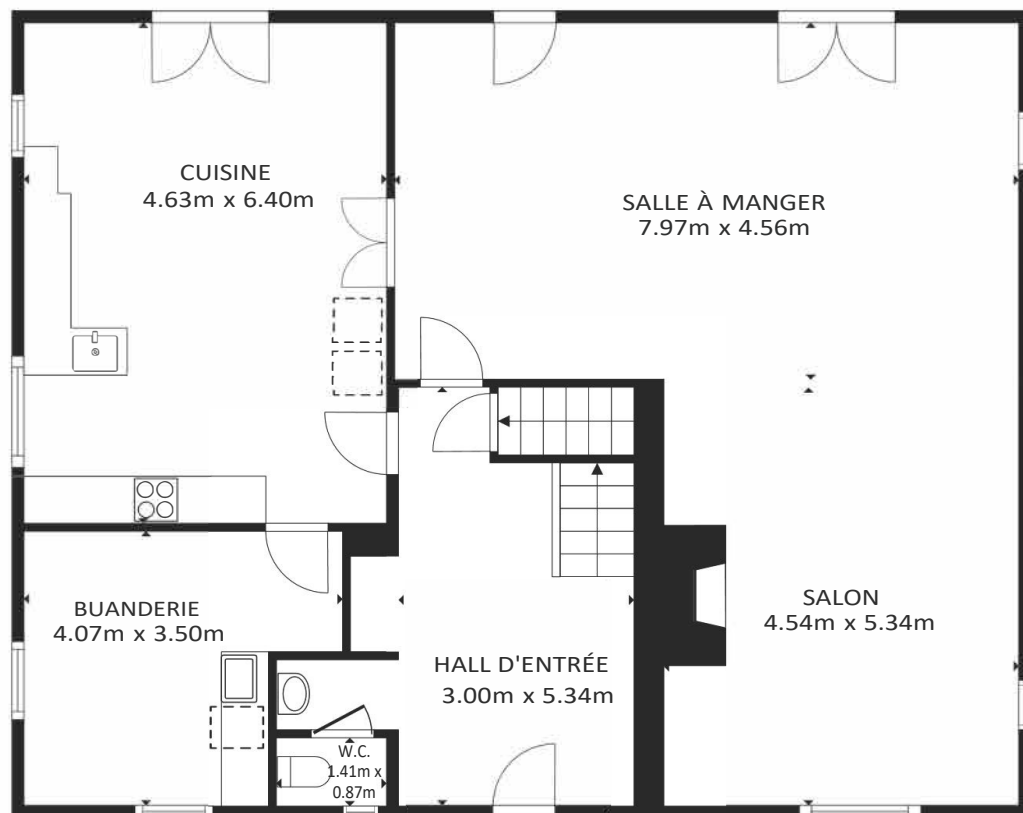
REZ-DE-CHAUSSEE
